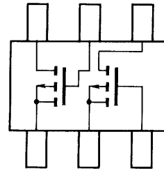
端子接続 (Top View)
