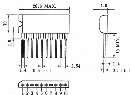
電極接続
