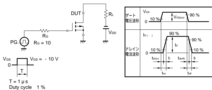
測定回路図2：スイッチングタイム測定回路
