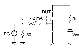
測定回路図3：ゲート電荷量測定回路
