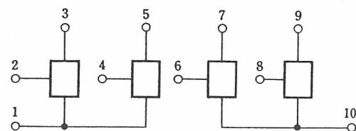
電極接続
