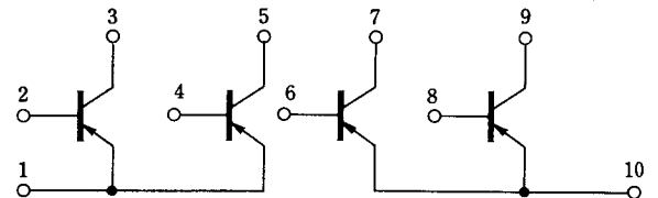
電極接続
