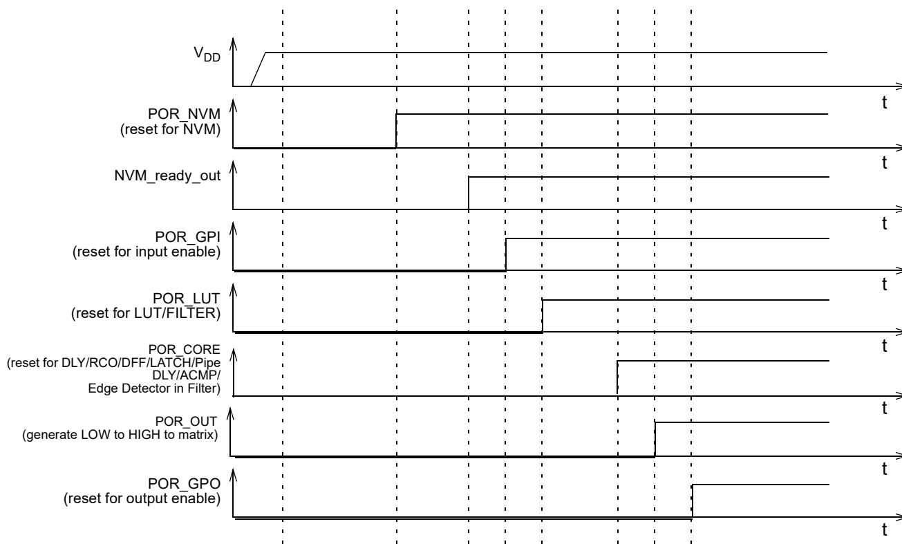
Figure 151. POR Sequence
