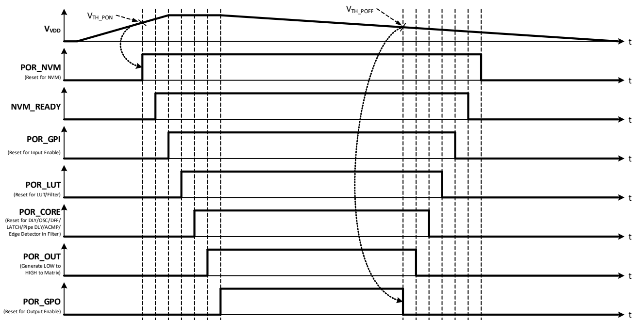
Figure 100. POR Sequence
