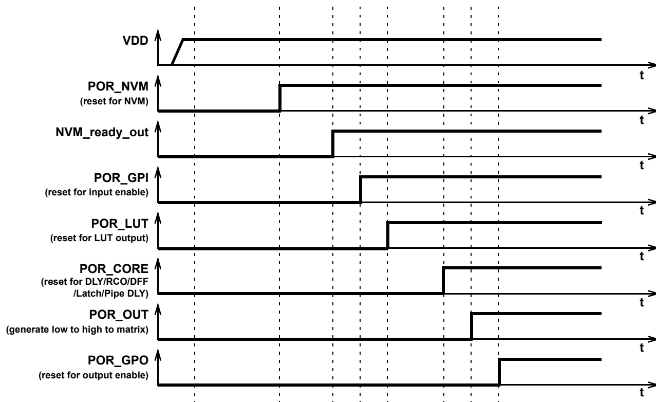
Figure 124. POR sequence
