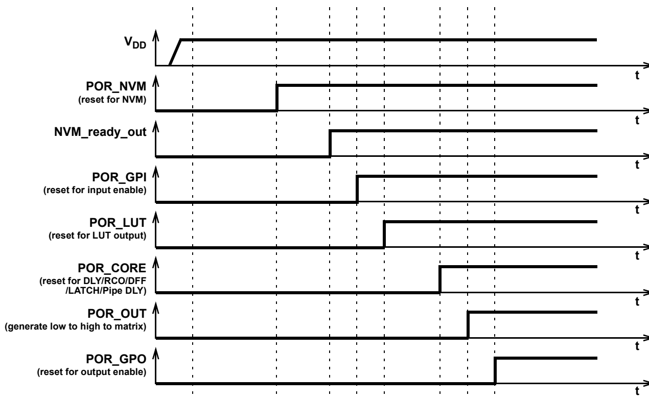
Figure 122. POR Sequence
