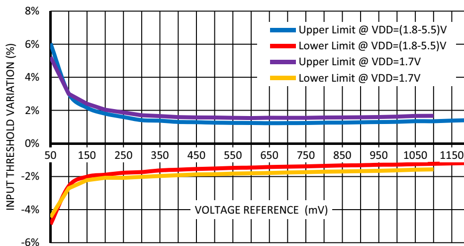
基準電圧に対する入力閾値電圧のばらつき範囲 (含 V_{\text{ref}} ばらつき、ACMP オフセット) (室温) LBW Mode – Disable, V_{\text{hys}}=0 mV.
