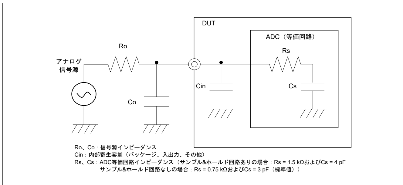
図 2.95 A/D コンバータの等価回路と周辺回路構成図
