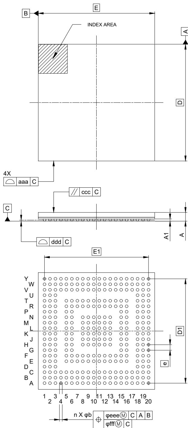
図 A1.1 320 ピン FBGA
