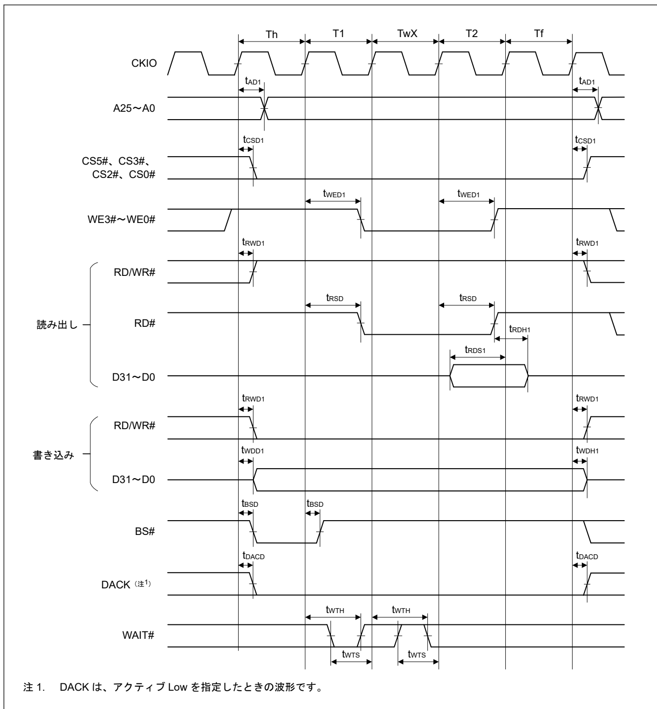
図 2.16 バイト選択付き SRAM バスサイクル (SW = 1 サイクル、HW = 1 サイクル、非同期外部ウェイト 1 挿入、BAS = 0 (ライトサイクル UB/LB 制御))
