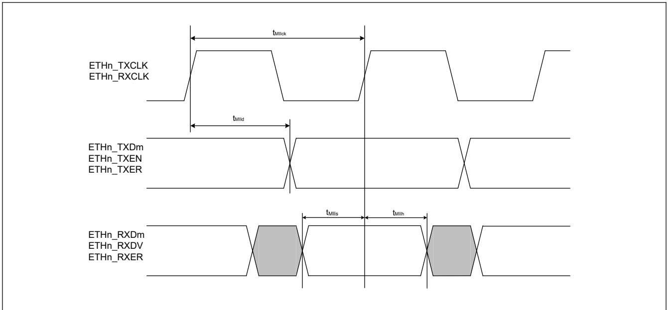
図 2.84 MII 送受信タイミング (n = 0~2, m = 0~3)
