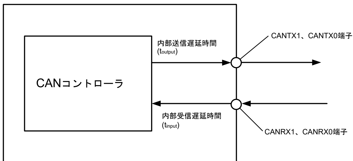
図 2.64 CAN インタフェース条件
