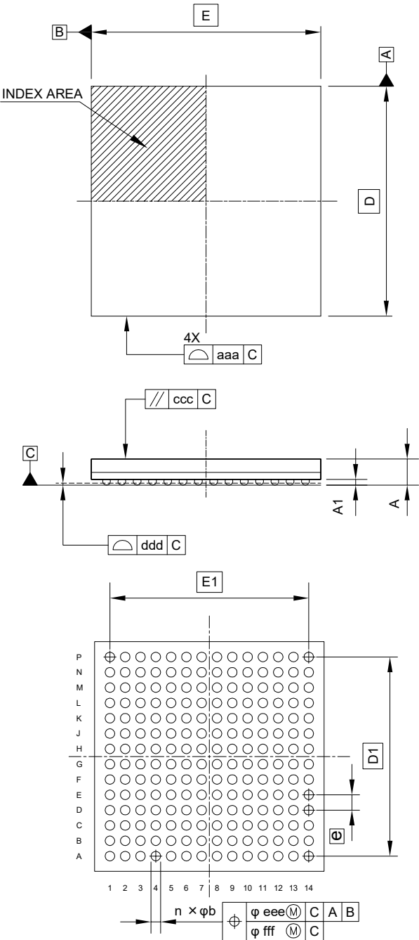
図 A1.1 196 ピン FBGA 0.8 mm ピッチ
