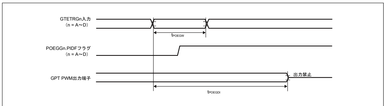
図 2.50 GTETRn 端子の入カレベル検出に対応した検出フラグによる POEG の出力禁止時間
