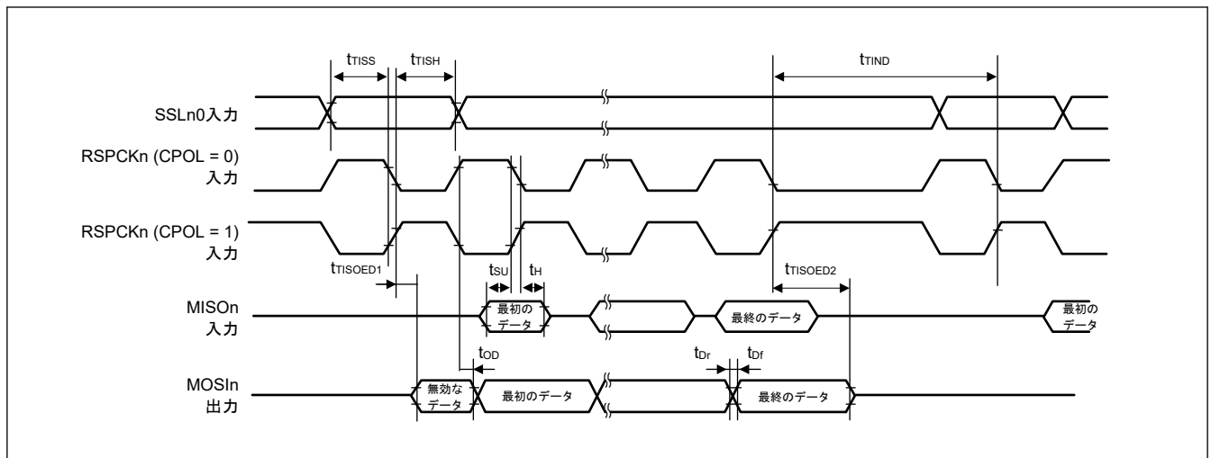
図 2.71 SPI タイミング (スレーブ、TI SSP、パースト転送時の遅延あり)
