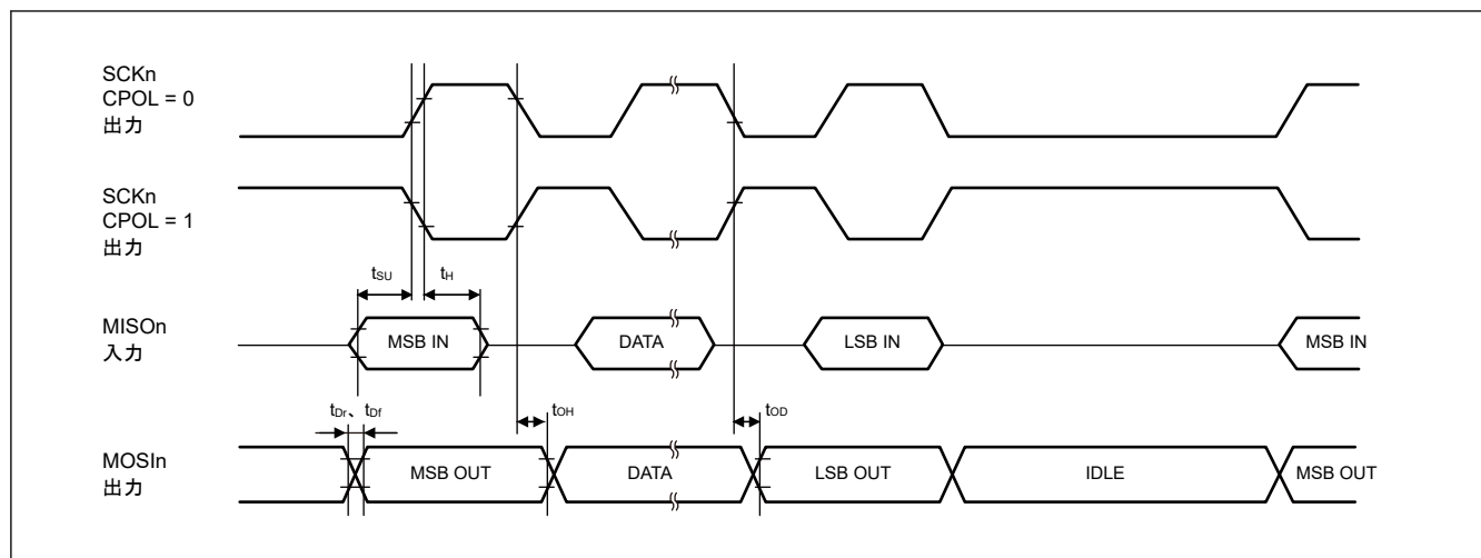
図 2.59 SCI 簡易 SPI モードタイミング (マスタ、CPHA = 0)
