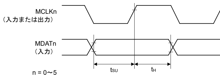
図 2.79 受信タイミング (MCLKn 立ち上がり同期)
