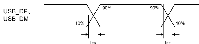
図 2.92 USB_DP、USB_DM の出カタイミング（フルスピード時）
