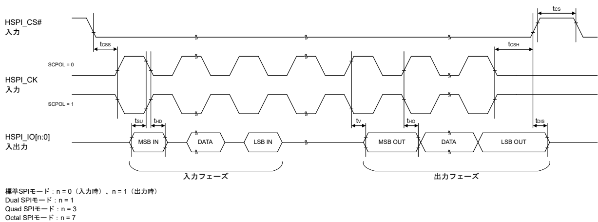
図 2.89 SHOSTIF タイミング (SCPH = 1)
