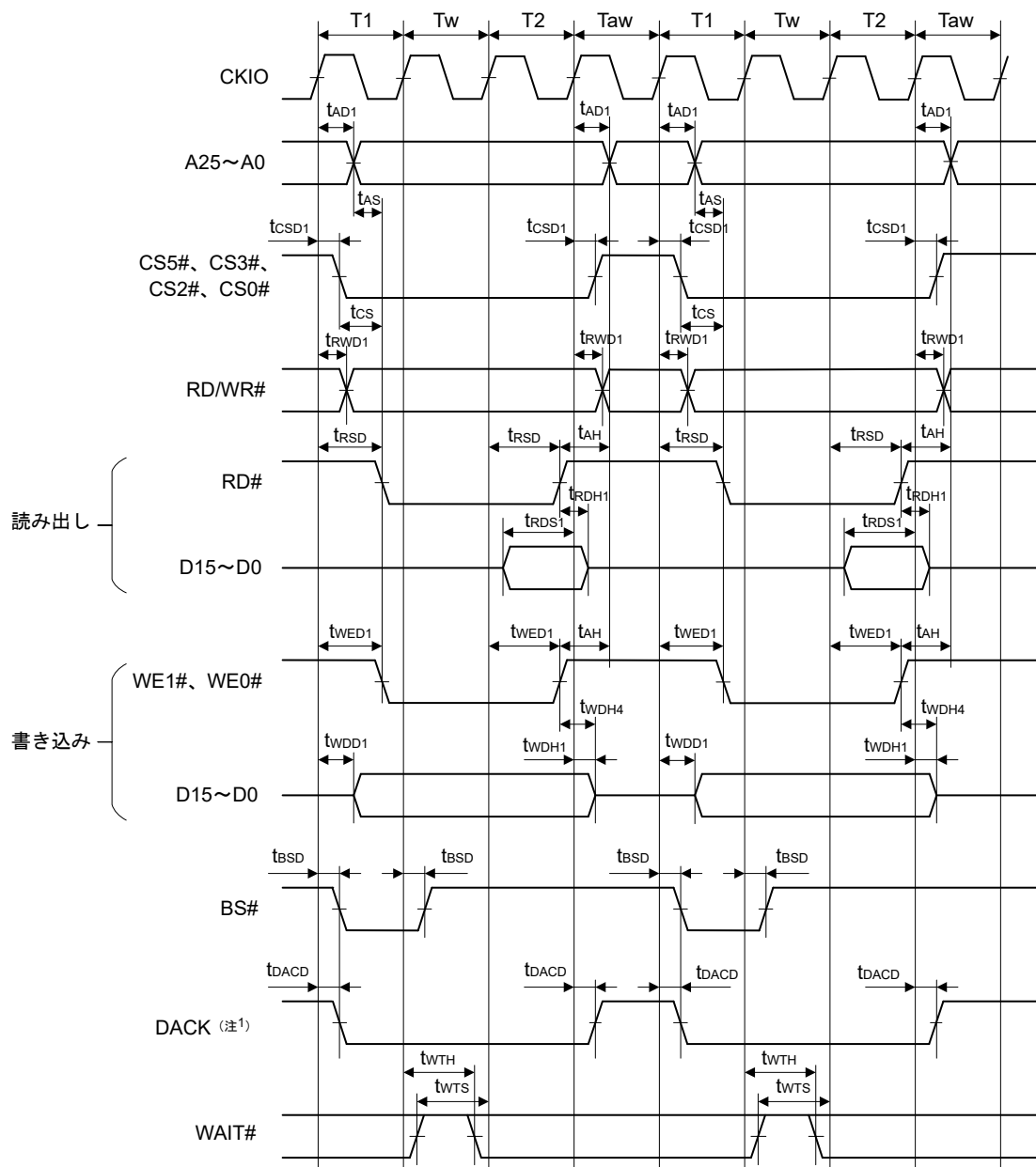
図 2.14 SRAM インタフェース基本バスサイクル (ソフトウェアウェイト 1、外部ウェイト有効 (WM = 0)、アイドルサイクルなし)
