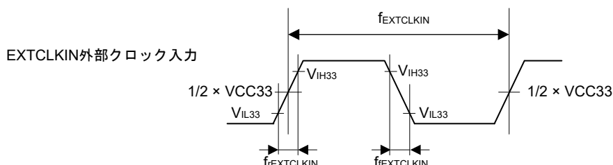
図 2.4 EXTCLKIN 外部クロック入力タイミング
