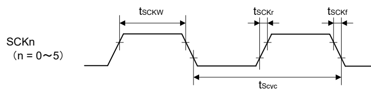
図 2.55 SCK クロック入出力タイミング
