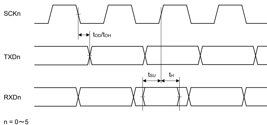
図 2.57 クロック同期式モードにおける SCI 入出力タイミング
