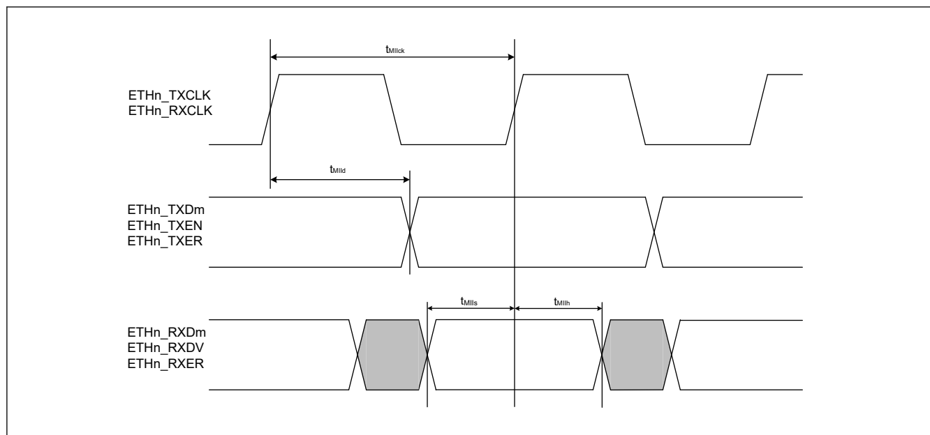
図 2.83 MII 送受信タイミング ( n = 0 \sim 2 , m = 0 \sim 3 )
