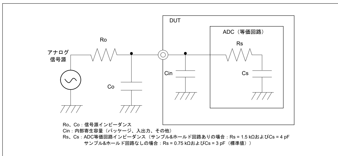
図 2.96 A/D コンバータの等価回路と周辺回路構成図
