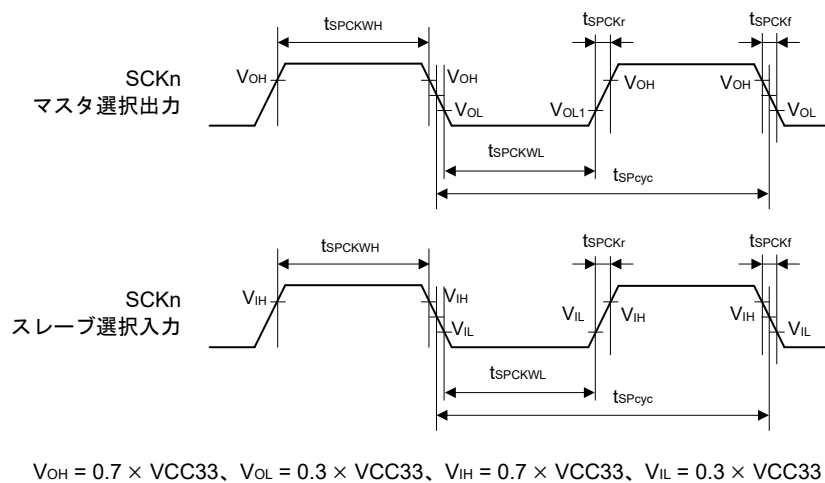
図 2.58 SCI 簡易 SPI モードクロックタイミング
