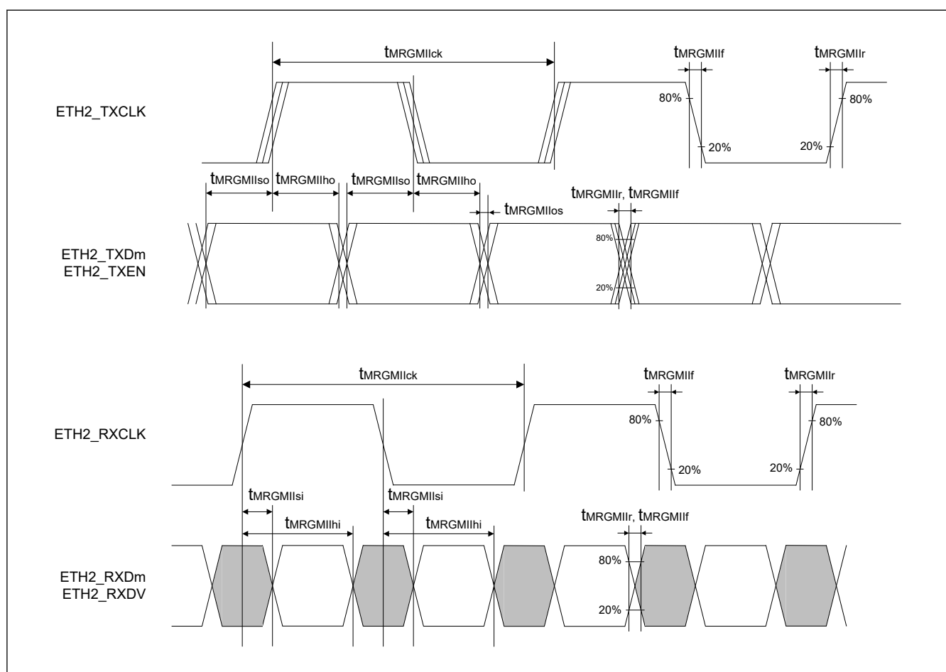
図 2.84 RGMII 送受信タイミング (MAC-to-MAC 接続モード) ( m = 0 \sim 3 )
