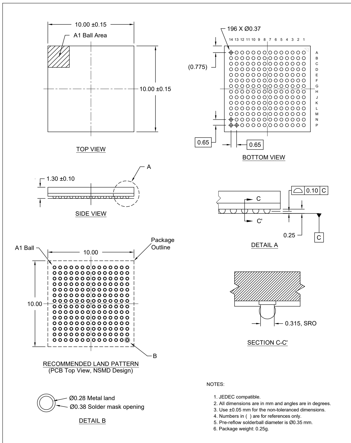
図 A1.2 196 ピン BGA 0.65 mm ピッチ
