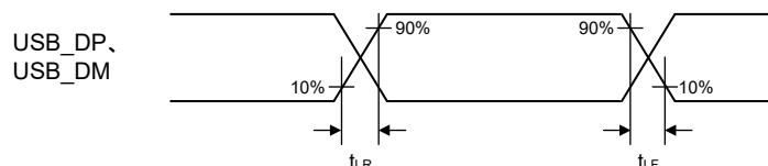
図 2.90 USB_DP、USB_DM の出カタイミング（ロースピード時／ホストのみ）
