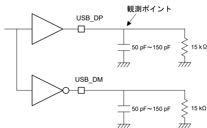
図 2.91 測定回路（ロースピード時／ホストのみ）
