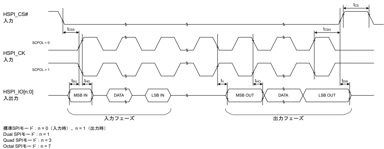
図 2.88 SHOSTIF タイミング (SCPH = 0)
