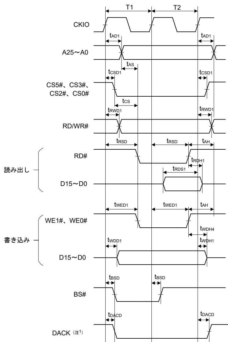
図 2.11 SRAM インタフェース基本バスサイクル (ウェイトなし)
