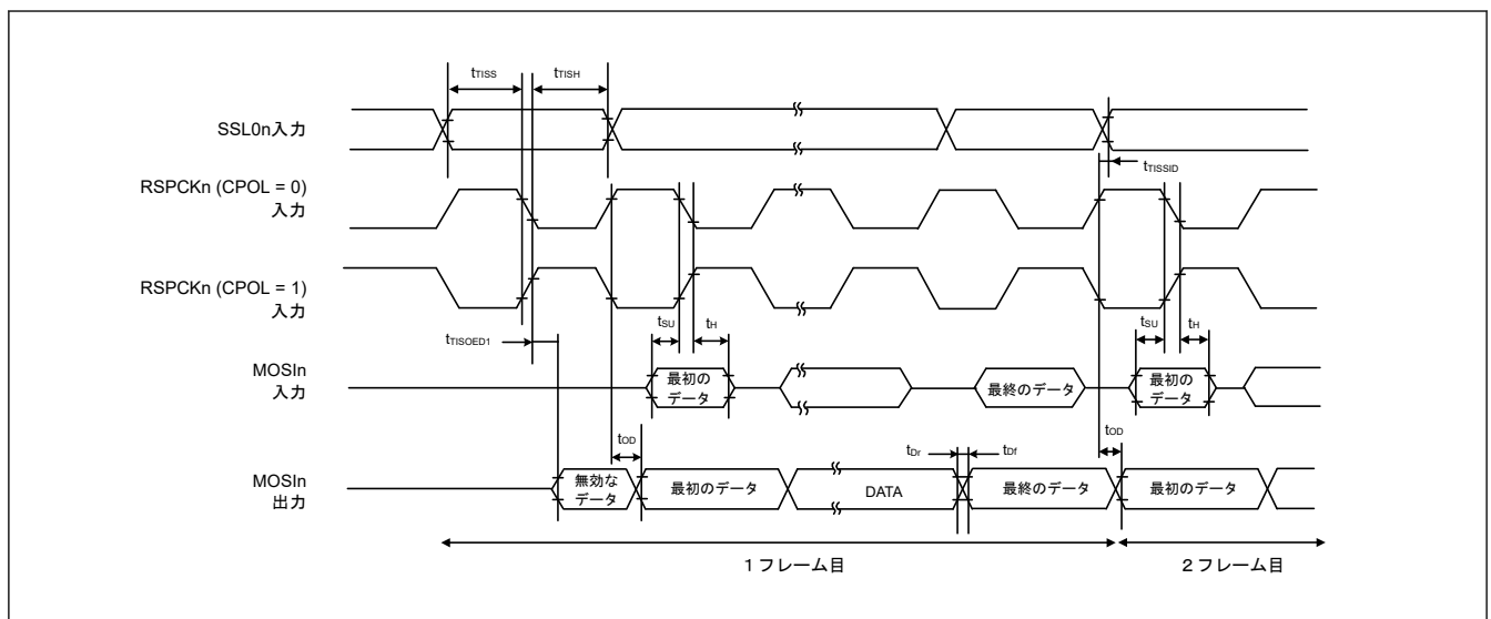
図 2.72 SPI タイミング (スレーブ、TI SSP、パースト転送時の遅延なし)
