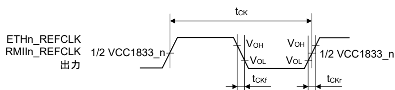
図 2.3 イーサネット PHY 基準クロック出力タイミング
