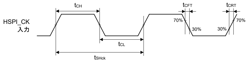
図 2.87 SHOSTIF クロックタイミング
