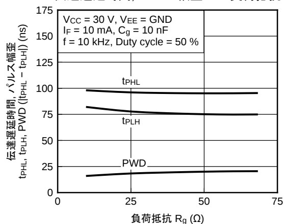
伝達遅延時間, パルス幅歪 vs. 負荷抵抗
