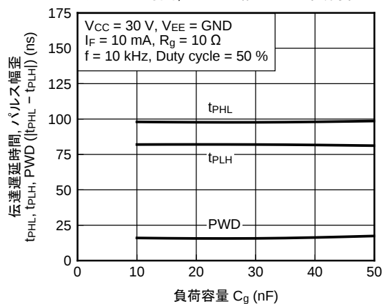
伝達遅延時間, パルス幅歪 vs. 負荷容量
