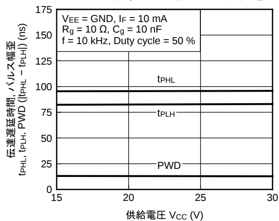
伝達遅延時間, パルス幅歪 vs. 供給電圧
