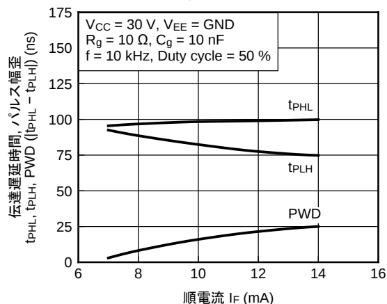
伝達遅延時間, パルス幅歪 vs. 順電流
