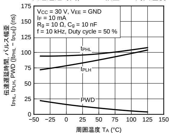
伝達遅延時間, パルス幅歪 vs. 周囲温度
