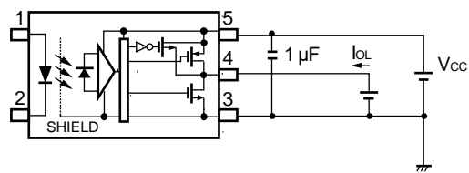
図4 V OL 測定回路
