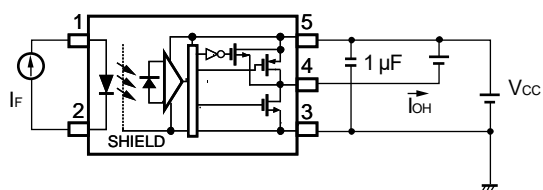
図3 V OH 測定回路
