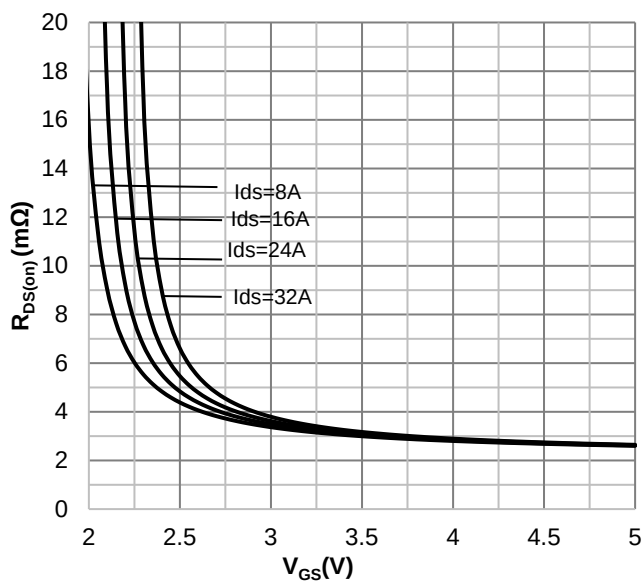
Figure 4. R_{DS(on)} vs V_G , Parameter I_{DS}
