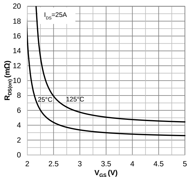
Figure 5. R_{DS(on)} vs V_G , Parameter T_J
