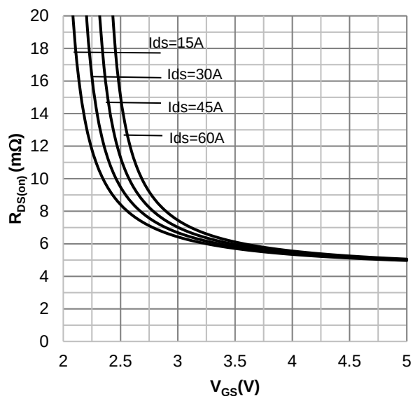
Figure 4. R_{DS(on)} vs V_G , Parameter I_{DS}
