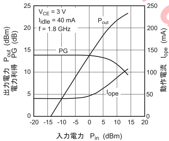
出力電力, 電力利得 対 入力電力
