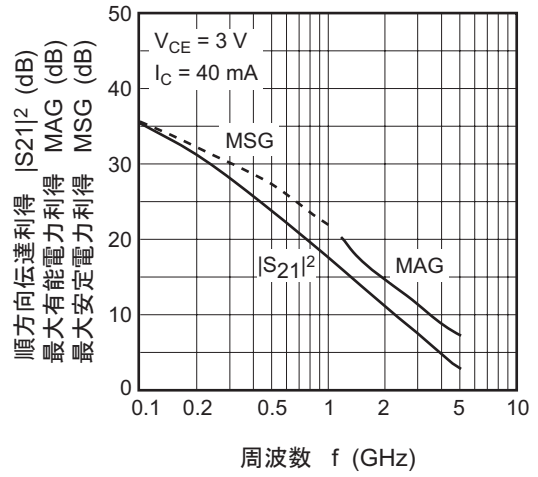
|S_{21}|^2 , MAG, MSG 対 周波数特性
