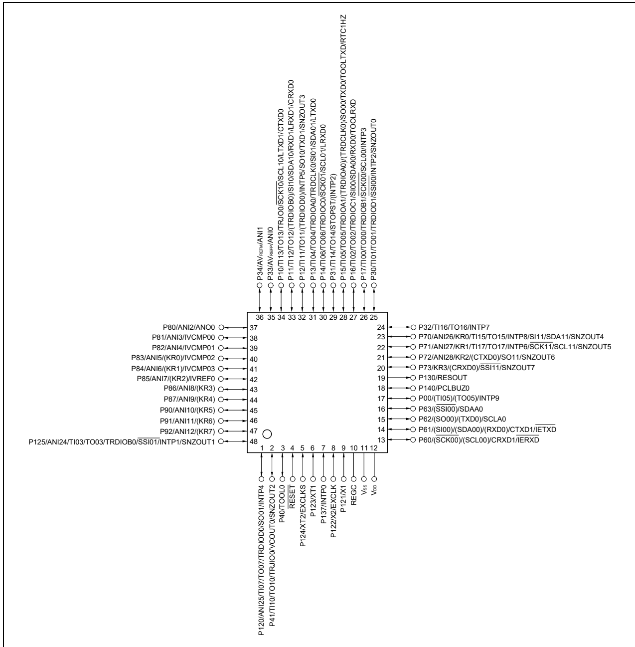
図1-10 RL78/F15の48ピン版の端子接続図
