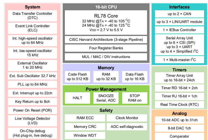
RL78/F15ブロック図
