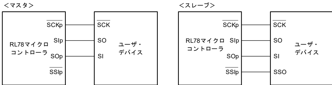
CSIモード接続図 (同電位通信時)
