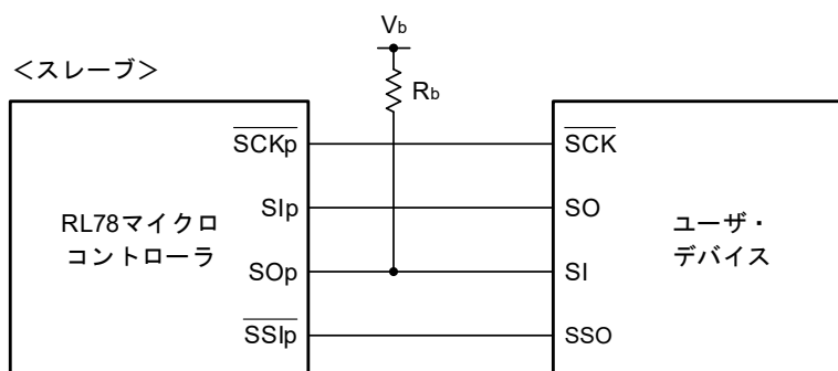
CSIモード接続図 (異電位通信時)
