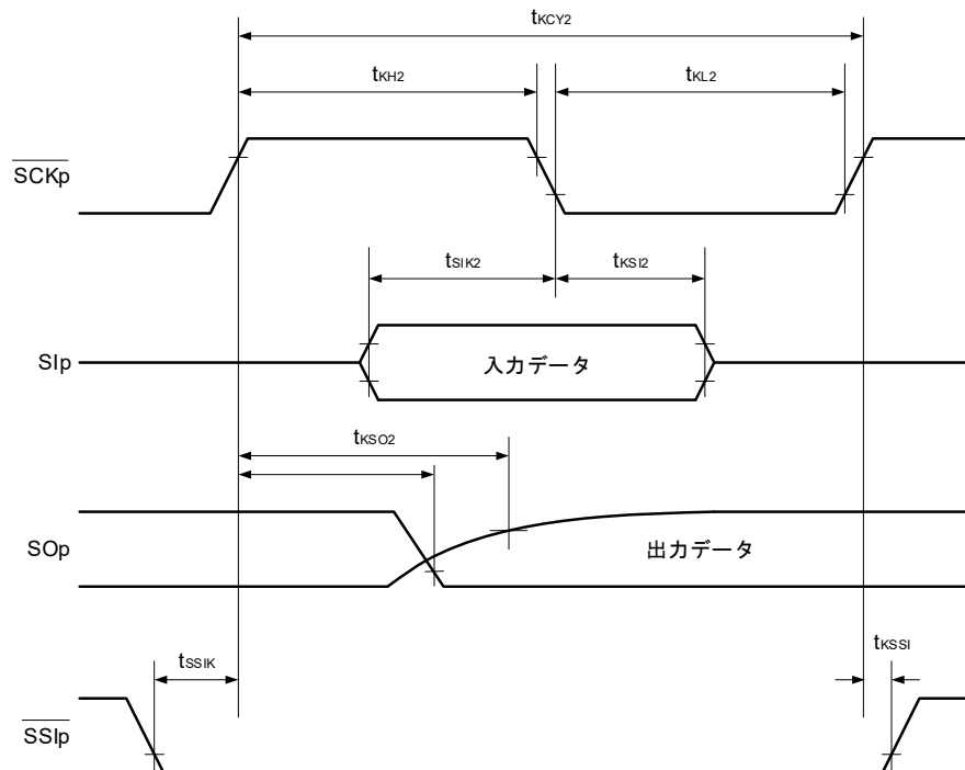
CSIモード・シリアル転送タイミング：スレーブ・モード（異電位通信時） （DAPmn = 0, CKPmn = 1またはDAPmn = 1, CKPmn = 0のとき）
