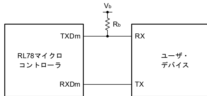
UARTモード接続図 (異電位通信時)
