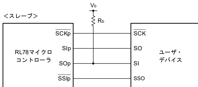
CSIモード接続図 (異電位通信時)
