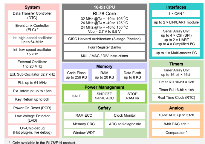
RL78/F13, F14ブロック図
