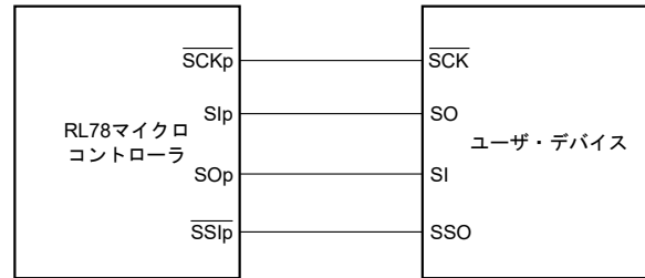
CSIモード接続図 (同電位通信時)
