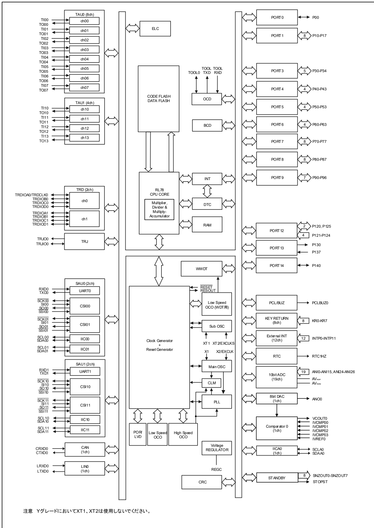
図1-6 機能ブロック図
