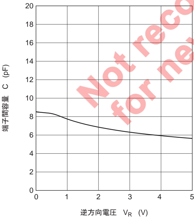
図3. 端子間容量 対 逆電圧特性
