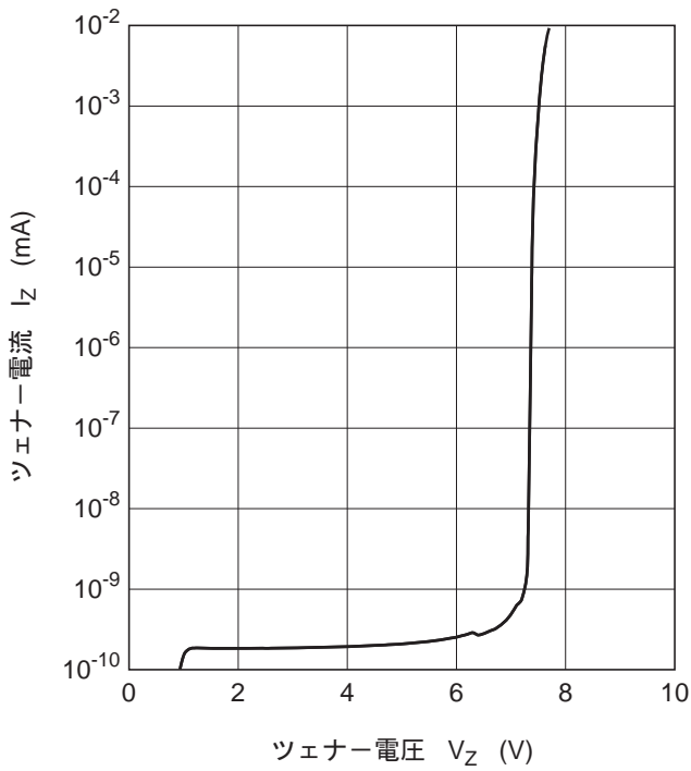
図1. ツェナー特性
