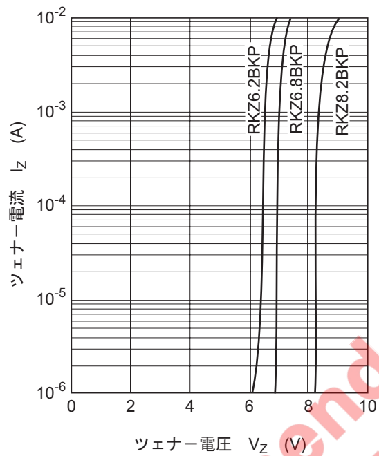
図1. ツェナー特性
