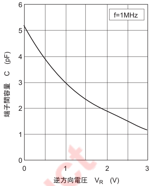
図2. 端子間容量 对 逆電圧特性
