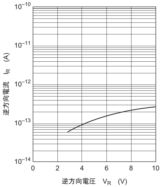
図1. 逆方向特性
