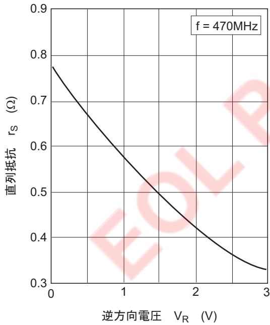
図3. 直列抵抗 对 逆電圧特性
