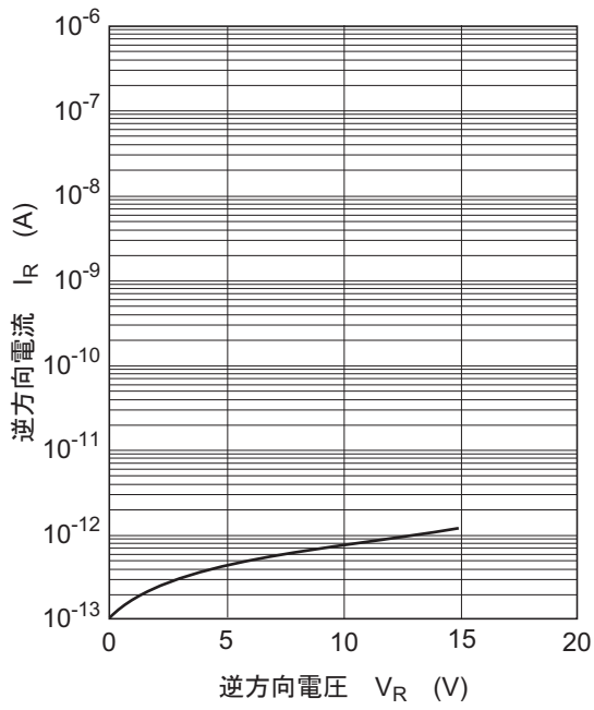
图1. 逆方向特性
