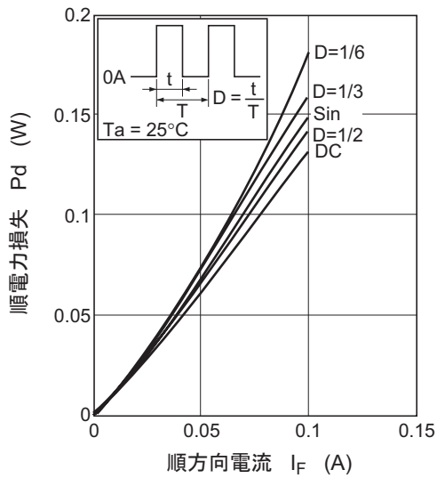
图4. 顺电力损失 对 顺电流特性
