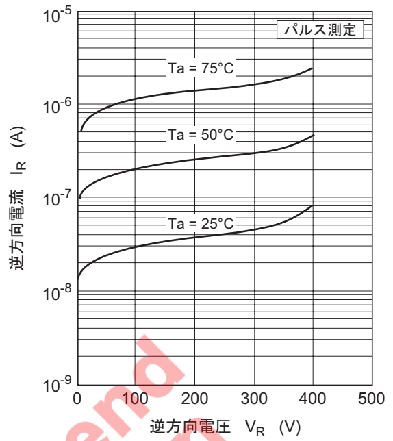
図2. 逆方向特性
