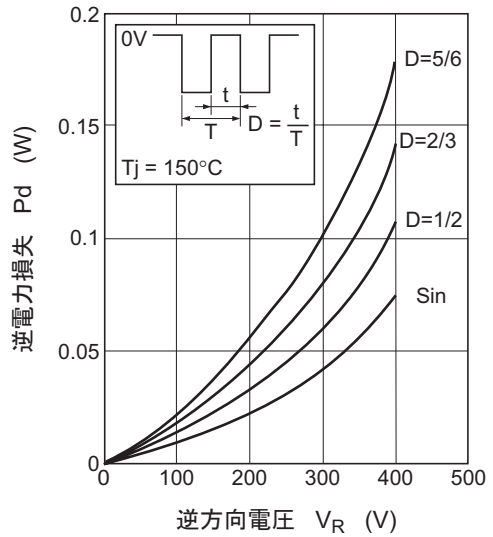
图5. 逆电力损失 对 逆电流特性
