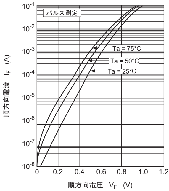
図1. 順方向特性
