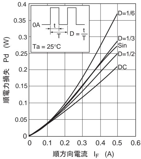
图4. 顺电力损失 对 顺电流特性
