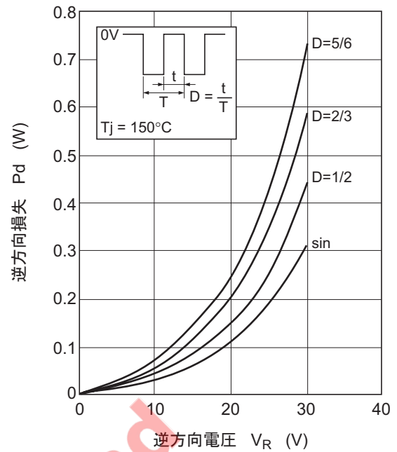
図5. 逆方向損失 対 逆方向電圧特性
