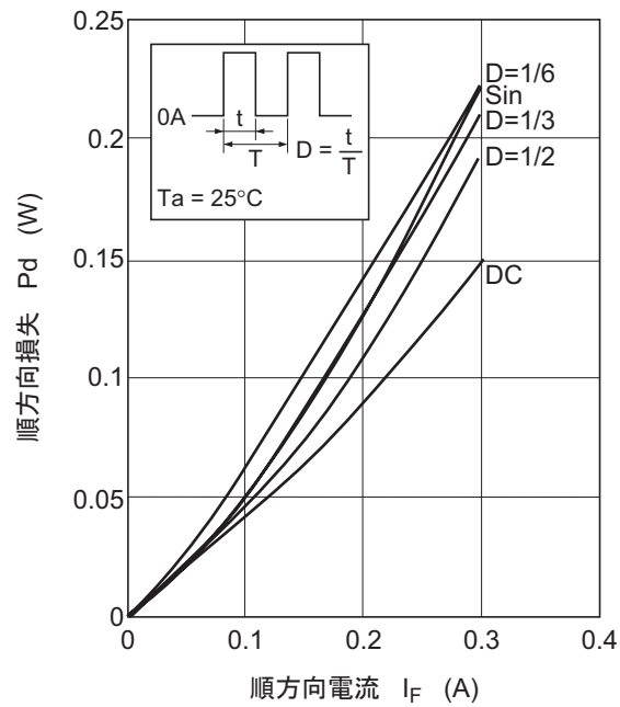
図4. 順方向損失 対 順方向電流特性
