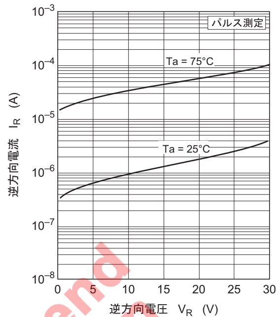
図2. 逆方向特性
