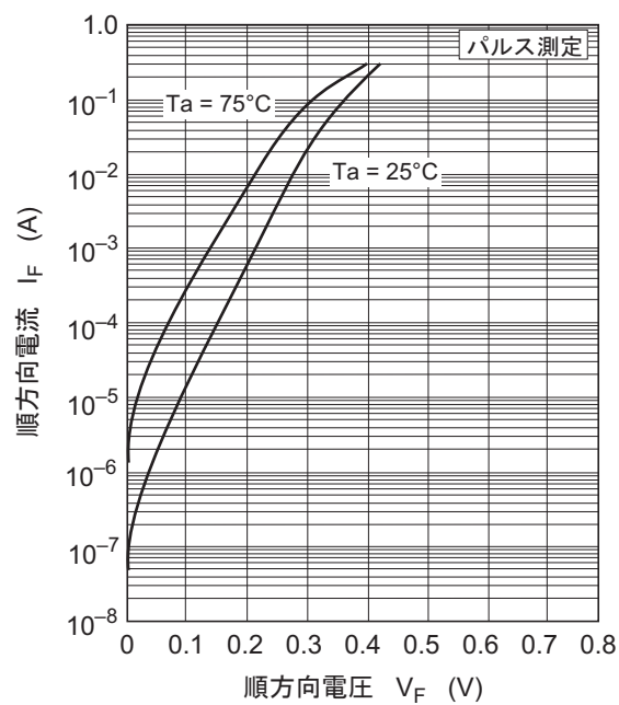
図1. 順方向特性
