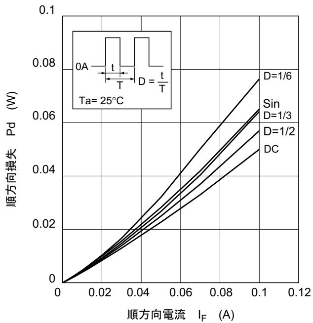
図4. 順方向損失 対 順電流特性
