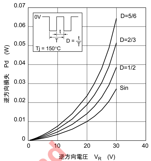
図5. 逆方向損失 対 逆電圧特性
