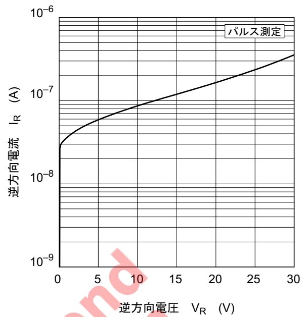
図2. 逆方向特性
