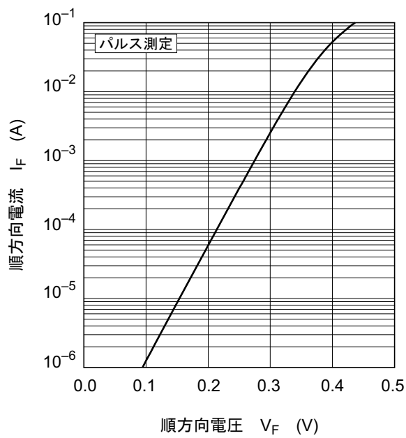
図1. 順方向特性
