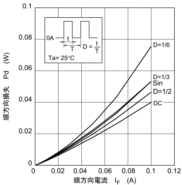
图4. 顺方向损失 对 顺电流特性
