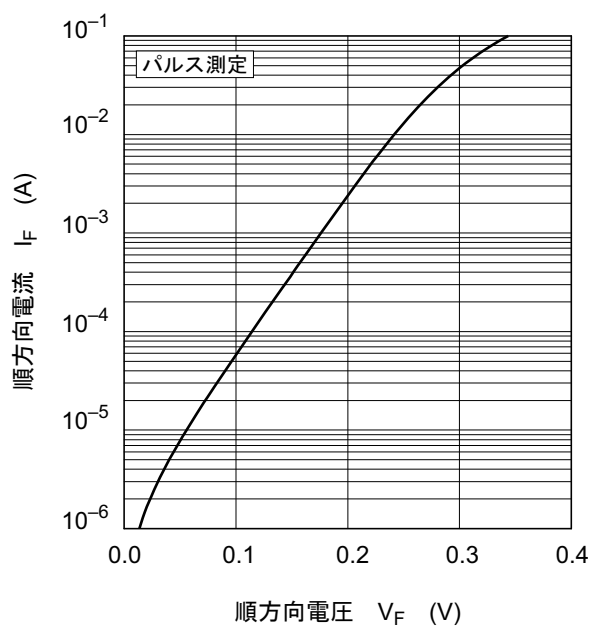
図1. 順方向特性
