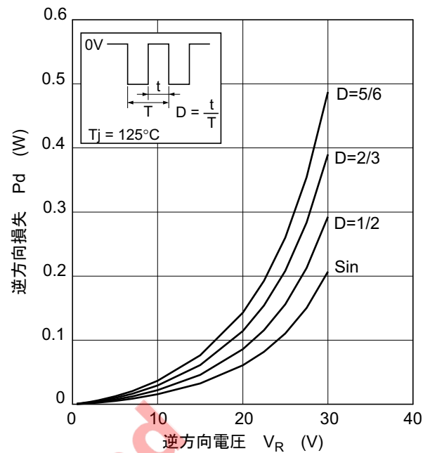
图5. 逆方向损失 对 逆电压特性
