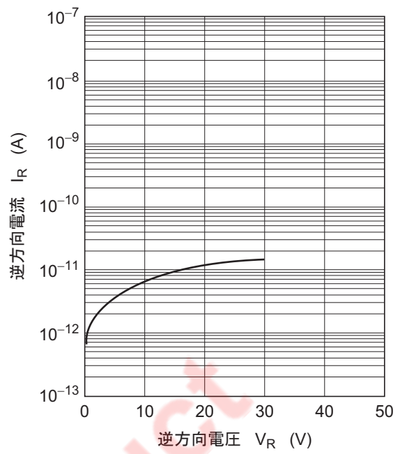
图2. 逆方向特性
