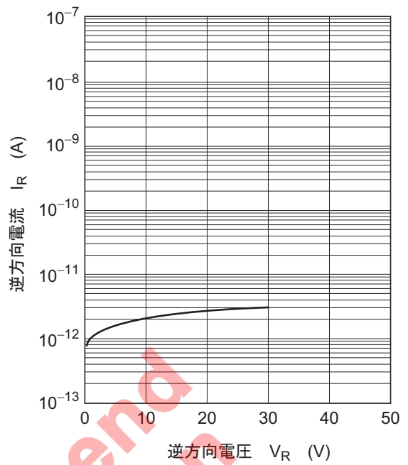
図2. 逆方向特性
