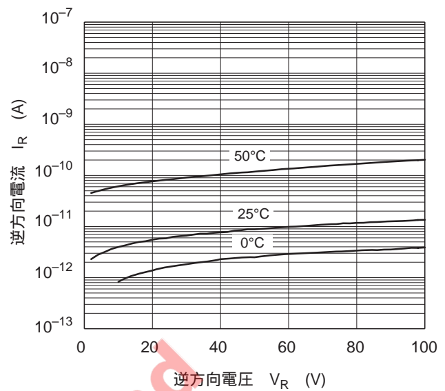
图2. 逆方向特性
