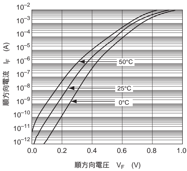
图1. 顺方向特性
