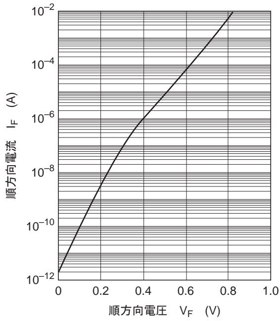
图1. 顺方向特性
