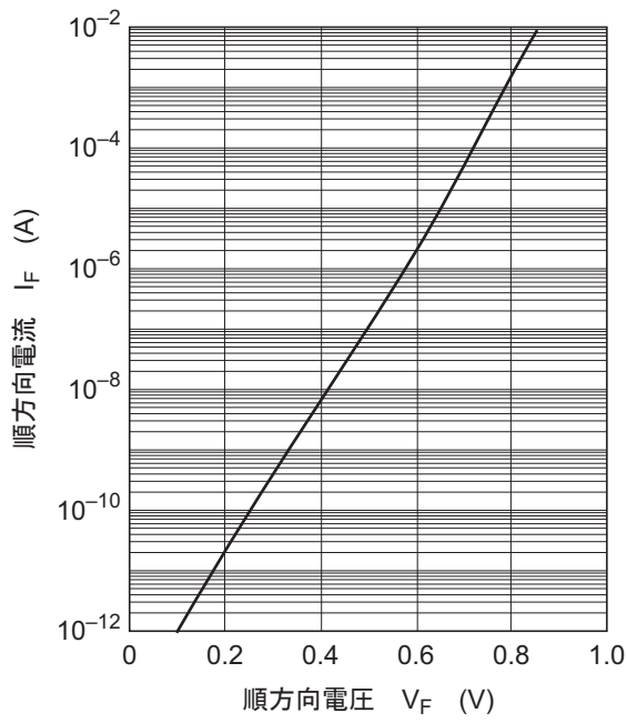
図1. 順方向特性
