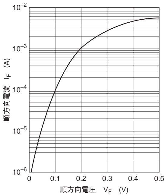
図1. 順方向特性
