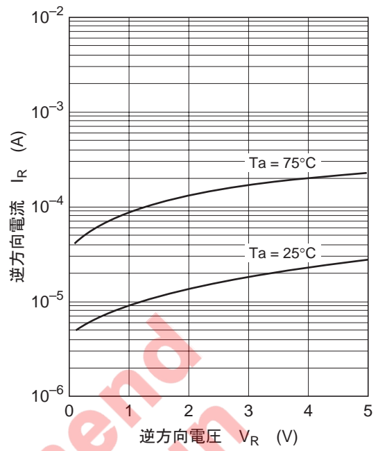
図2. 逆方向特性
