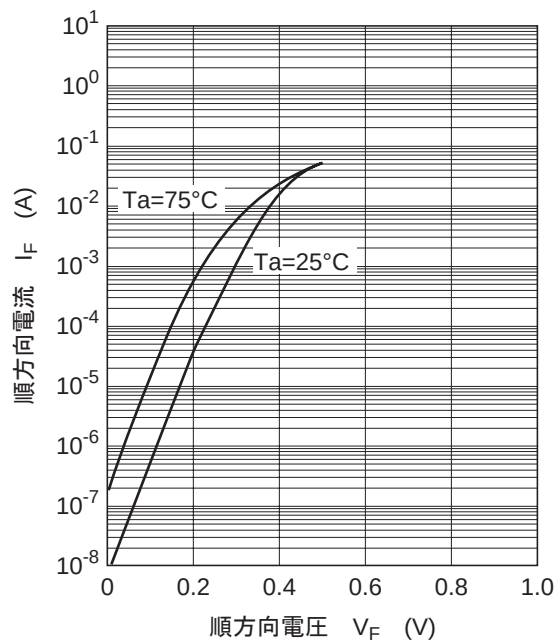
図1. 順方向特性
