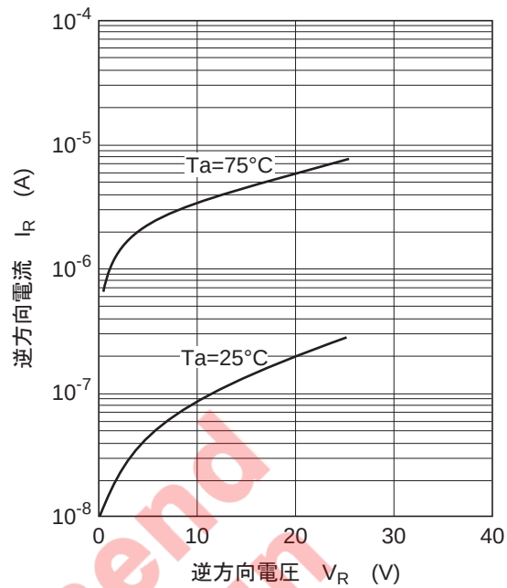
図2. 逆方向特性
