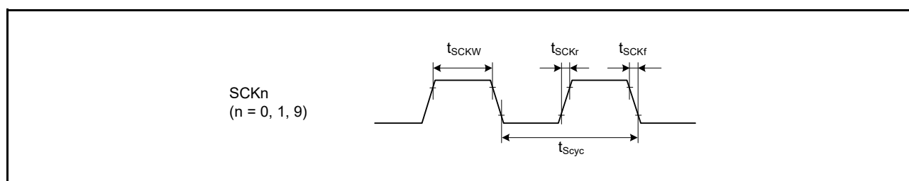
図 2.42 SCK クロック入カタイミング
