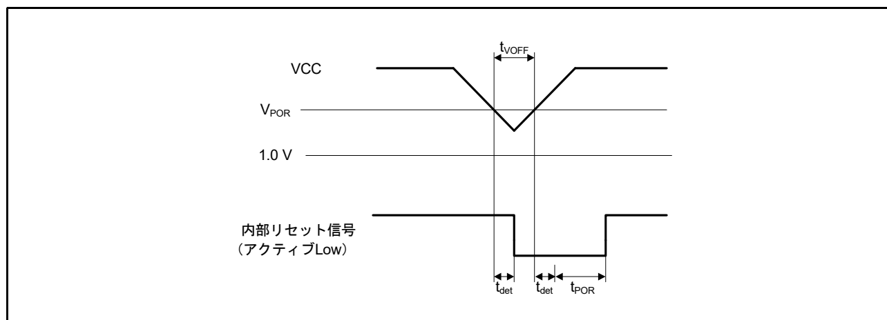
図 2.66 電圧検出しセットタイミング
