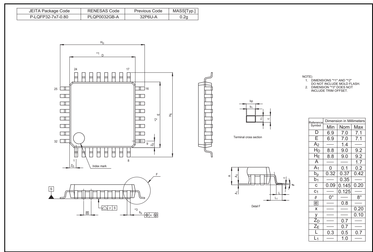
図 1.2 LQFP 32 ピン
