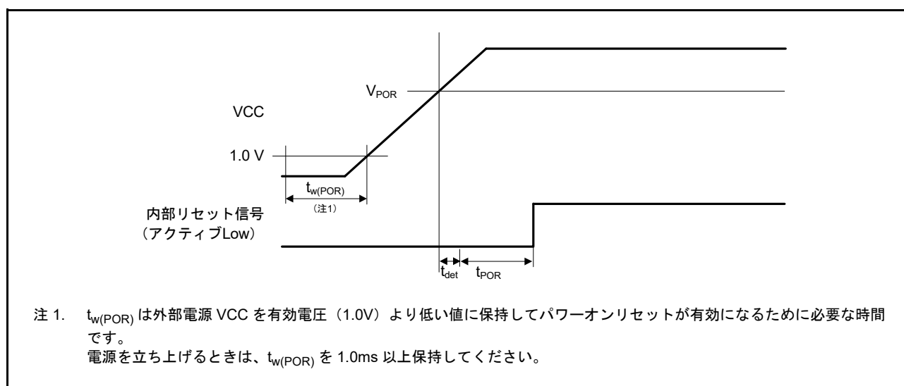
図 2.67 パワーオンリセットタイミング
