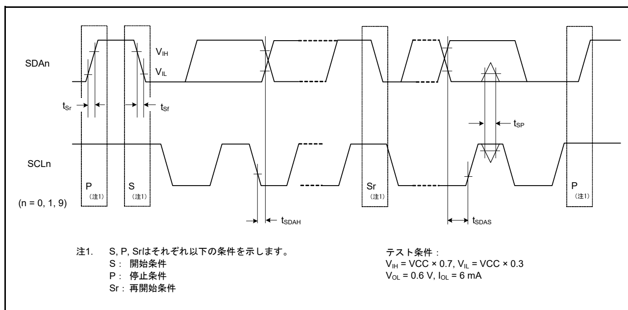
図 2.49 SCI 簡易 IIC モードタイミング
