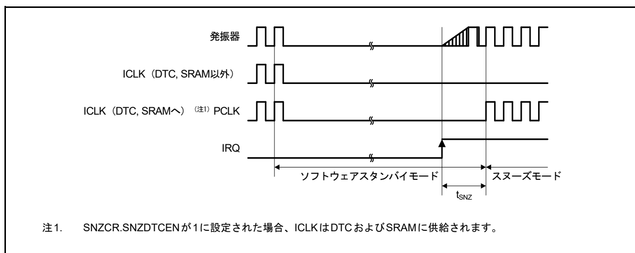
図 2.33 ソフトウェアスタンバイモードからスヌーズモードへの復帰タイミング
