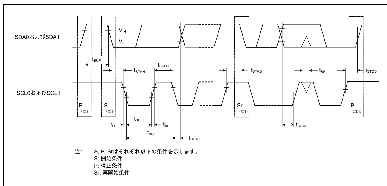
図 2.57 I 2 C バスインタフェース入出力タイミング
