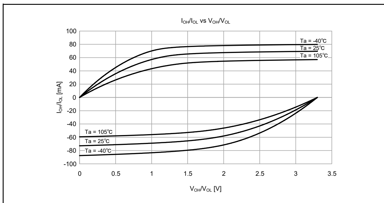
図 2.14 中駆動出力選択時の V_{CC} = 3.3\text{V} での V_{OH}/V_{OL} および I_{OH}/I_{OL} 温度特性 (参考データ)
