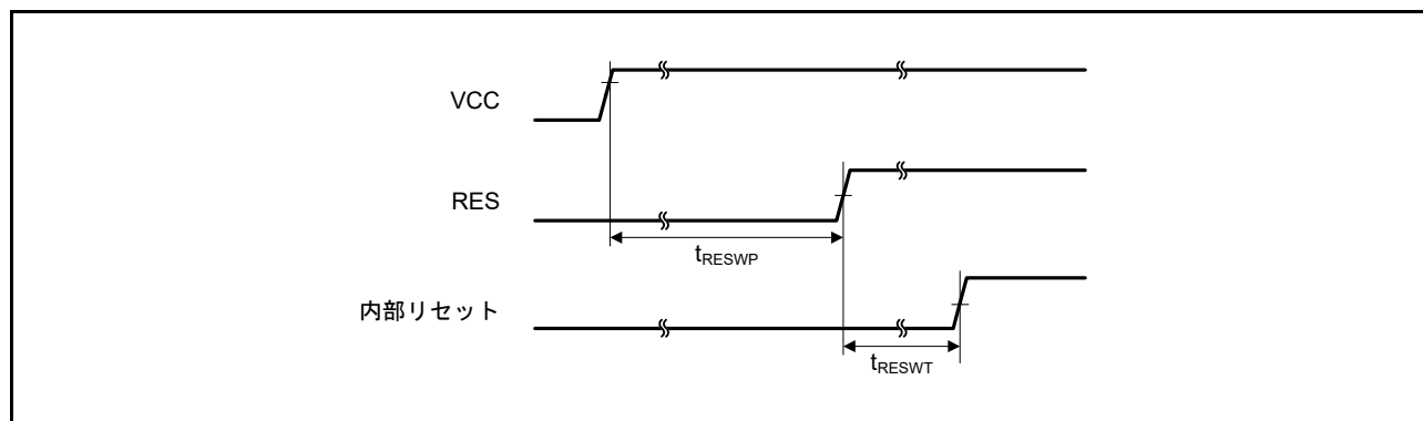
図 2.29 電源投入時リセット入力タイミグ
