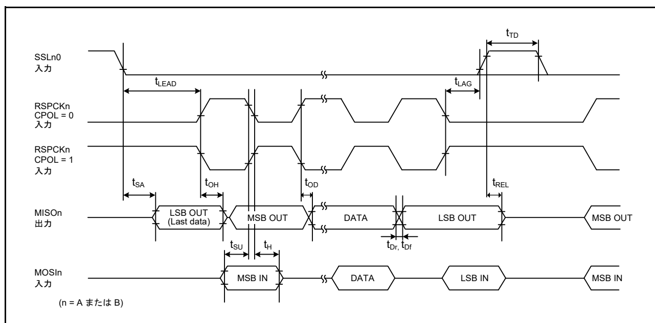
図 2.56 SPI タイミング (スレーブ、CPHA = 1)
