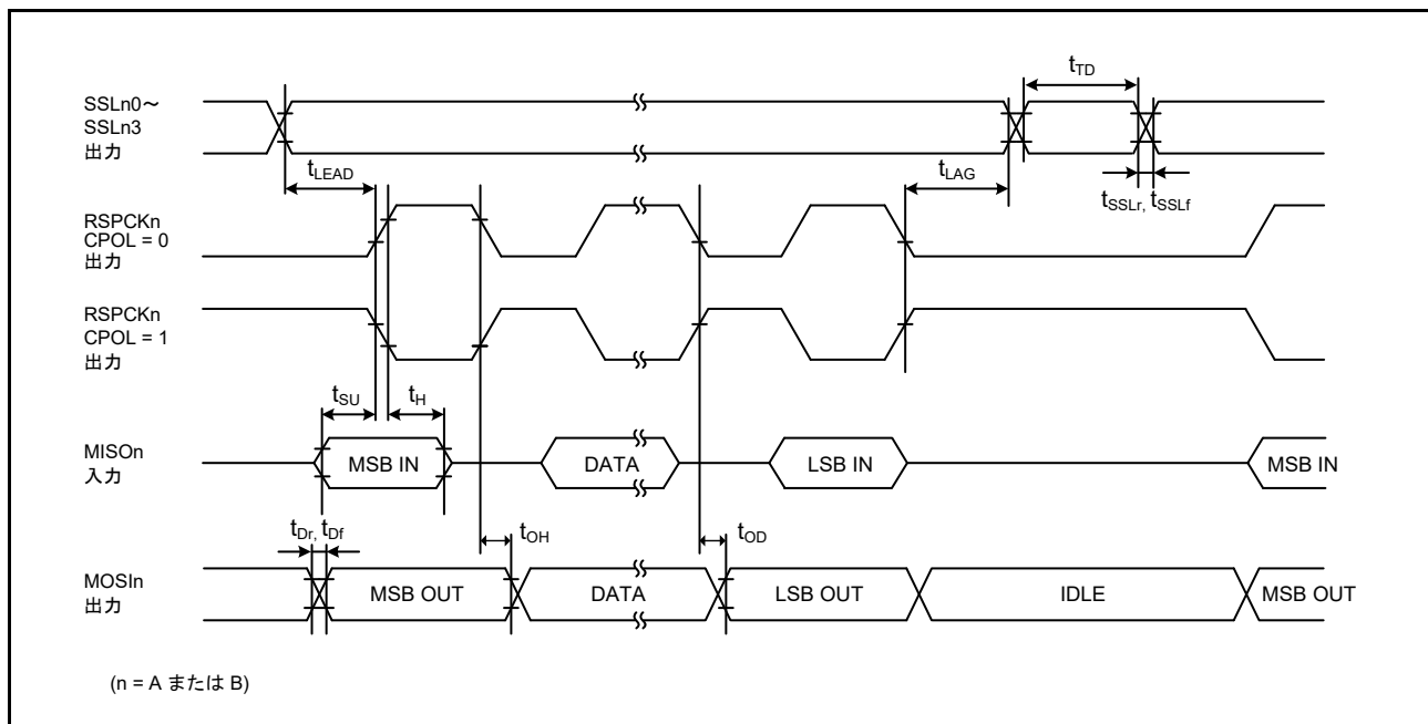
図 2.51 SPI タイミング (マスタ、CPHA = 0) (ビットレート : PCLKB を 2 分周以外に設定)
