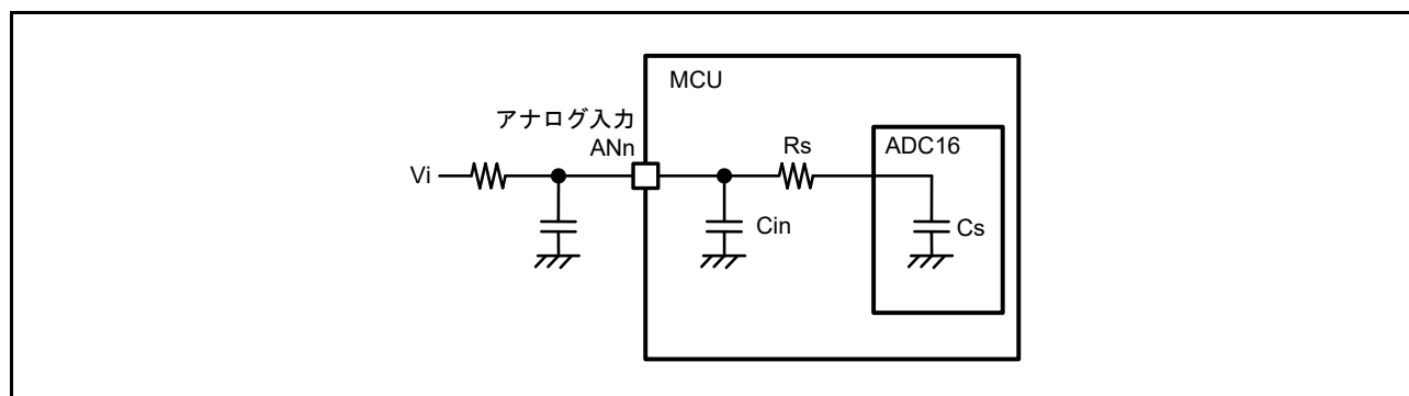
図 2.62 アナログ入力の等価回路
