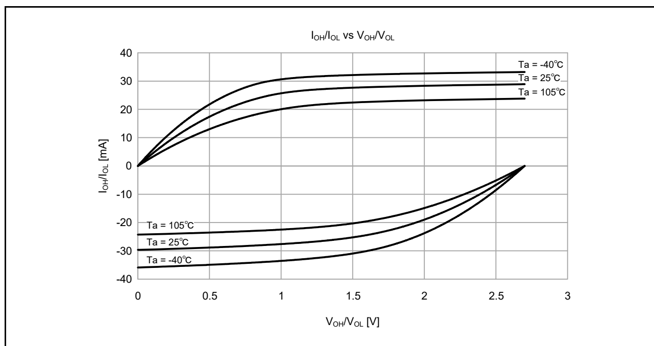
図 2.9 中駆動出力選択時の V_{CC} = 2.7\text{V} での V_{OH}/V_{OL} および I_{OH}/I_{OL} 温度特性（参考データ、P914 および P915 を除く）
