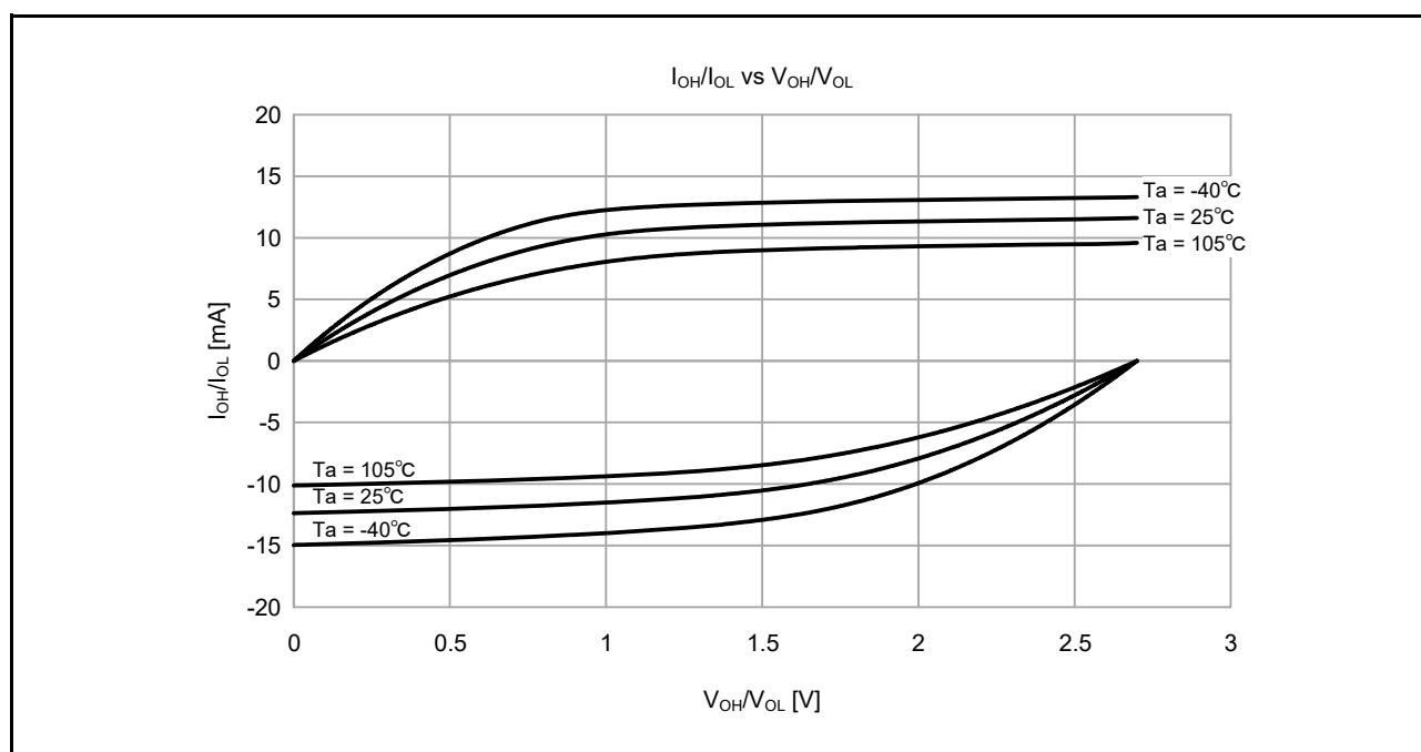
図 2.4 低駆動出力選択時の V_{CC} = 2.7\text{V} での V_{OH}/V_{OL} および I_{OH}/I_{OL} 温度特性（参考データ、P914 および P915 を除く）
