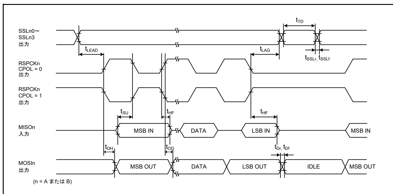
図 2.54 SPI タイミング (マスタ、CPHA = 1) (ビットレート : PCLKB を 2 分周に設定)
