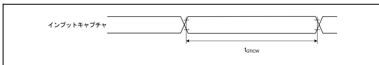
図 2.38 GPT インプットキャプチャタイミング
