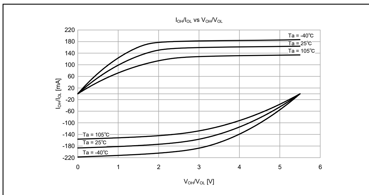
図 2.15 中駆動出力選択時の V_{CC} = 5.5\text{V} での V_{OH}/V_{OL} および I_{OH}/I_{OL} 温度特性 (参考データ)
