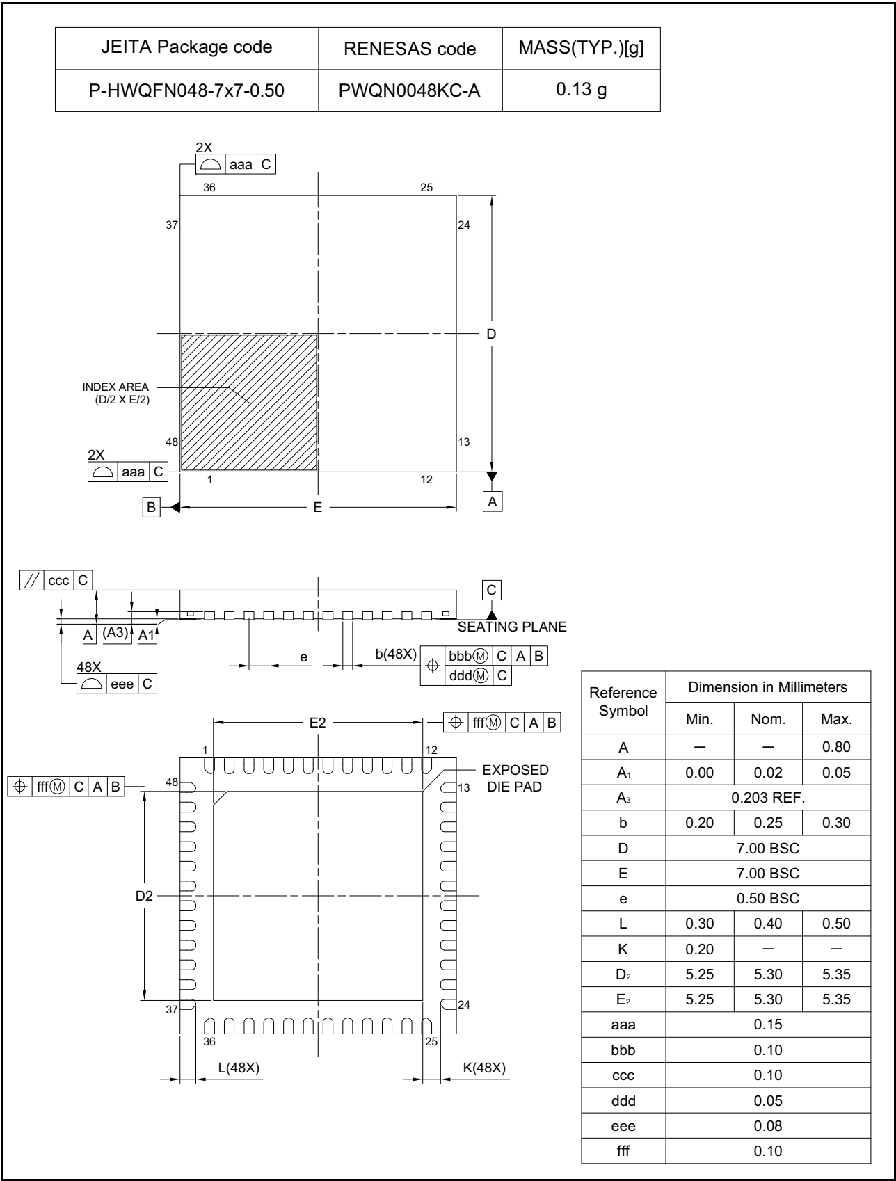
図 1.5 QFN48 ピン (2)
