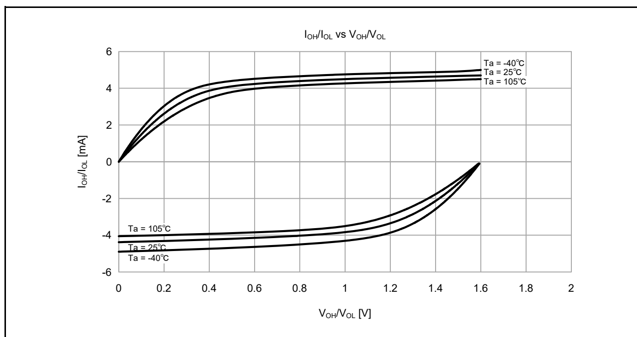
図 2.8 中駆動出力選択時の V_{CC} = 1.6\text{V} での V_{OH}/V_{OL} および I_{OH}/I_{OL} 温度特性（参考データ、P914 および P915 を除く）
