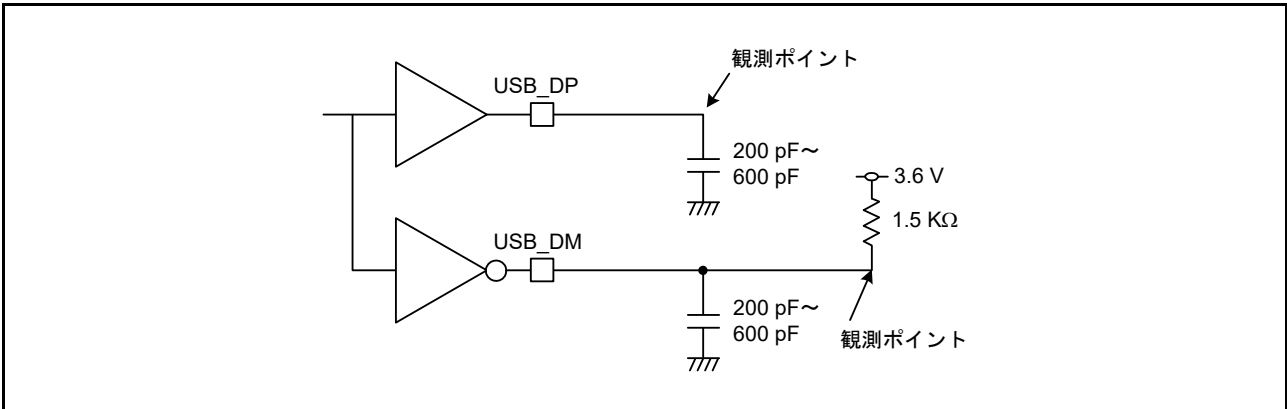
図 2.61 ロースピード (LS) 接続の測定回路
