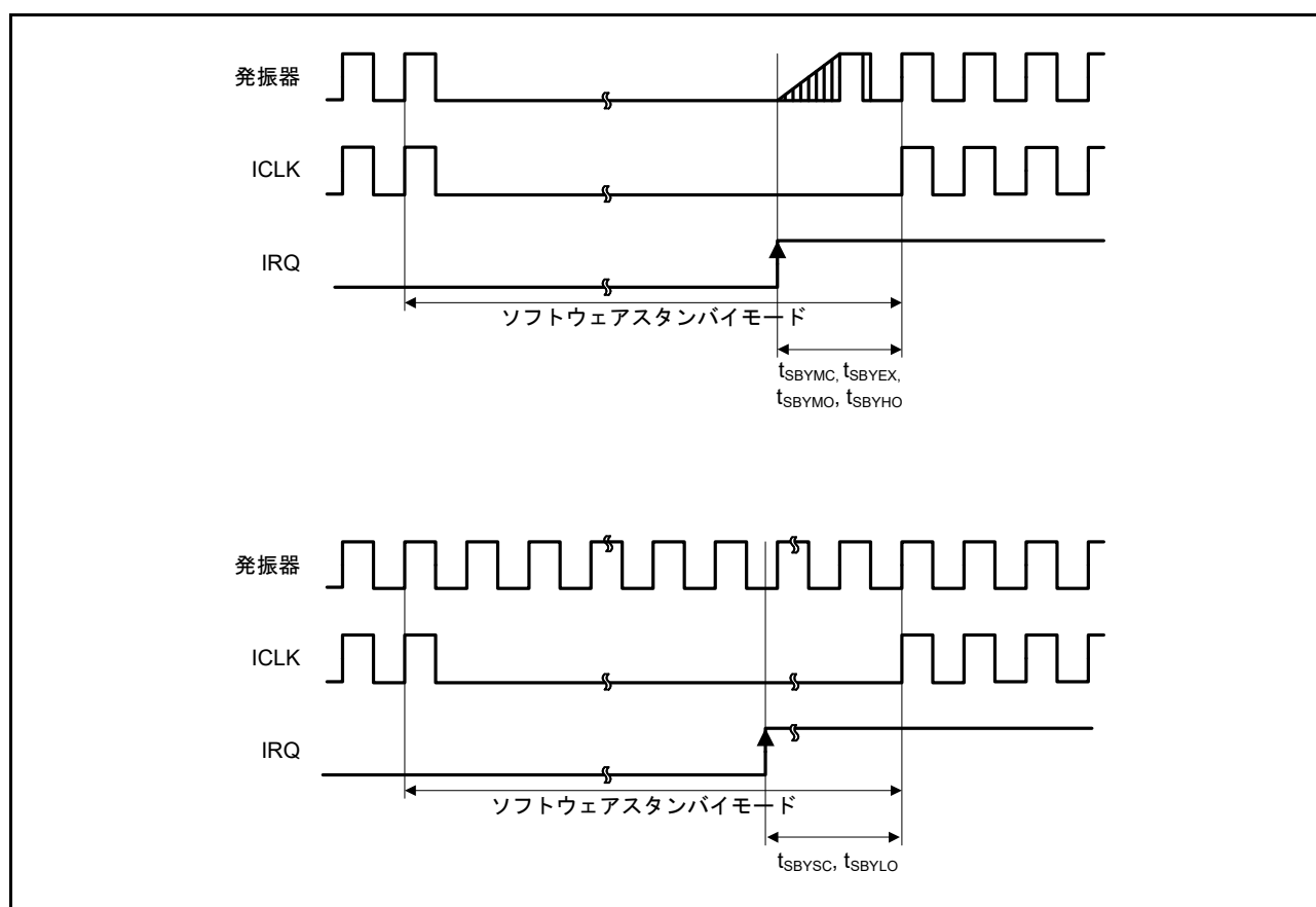
図 2.32 ソフトウェアスタンバイモード解除タイミング
