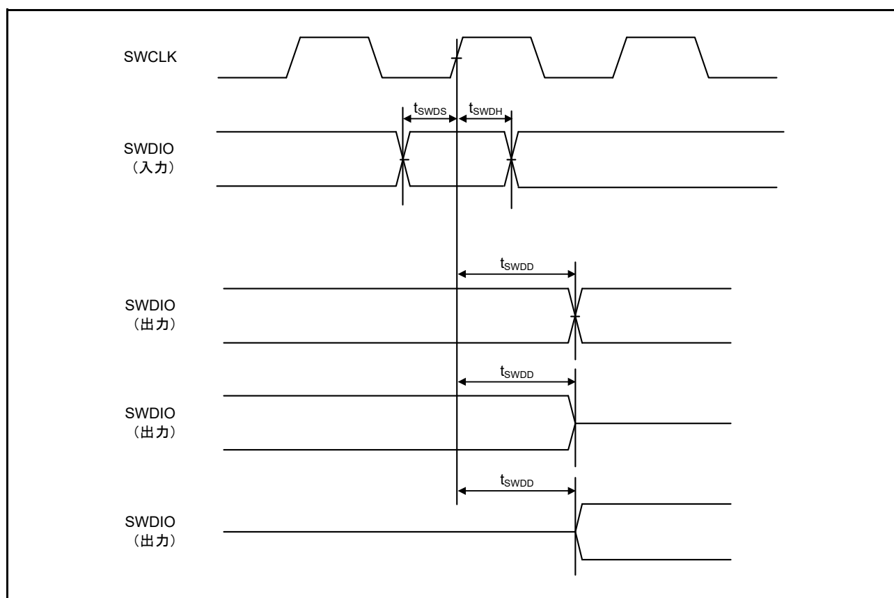
図 2.72 SWD 入出力タイミング
