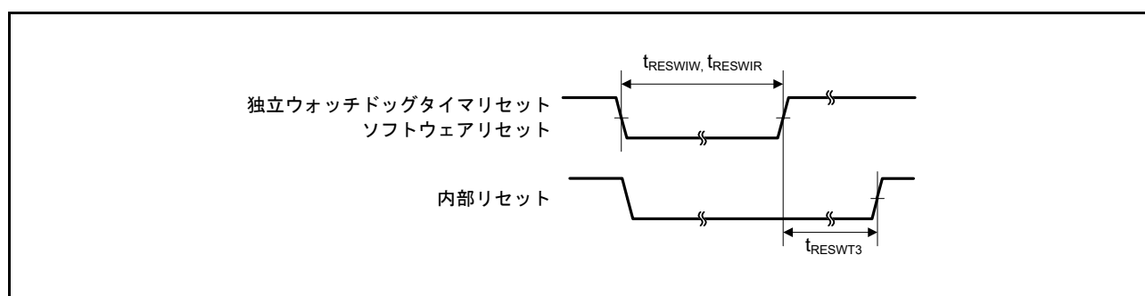
図 2.31 リセット入力タイミング (2)
