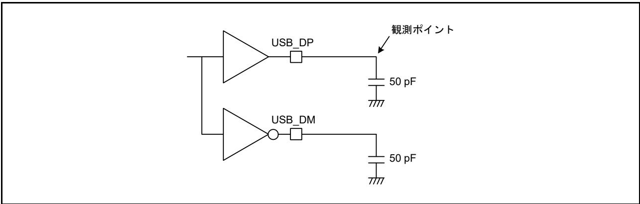
図 2.60 フルスピード (FS) 接続の測定回路
