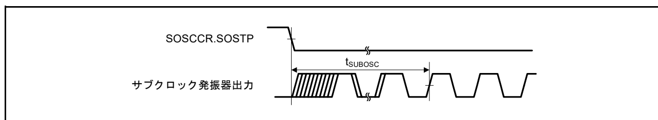
図 2.28 サブクロック発振開始タイミング
