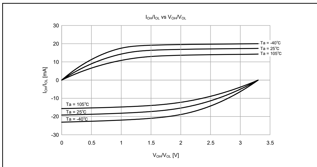
図 2.5 低駆動出力選択時の V_{CC} = 3.3\text{V} での V_{OH}/V_{OL} および I_{OH}/I_{OL} 温度特性（参考データ、P914 および P915 を除く）
