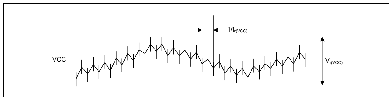
図 2.24 リップル波形
