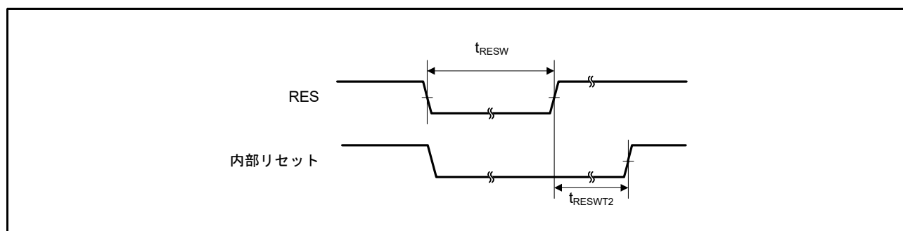
図 2.30 リセット入力タイミグ (1)
