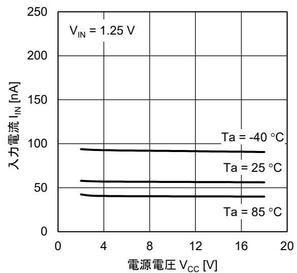
入力電流 - 電源電圧特性
