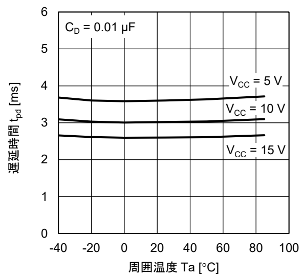
遅延時間 - 周囲温度特性
