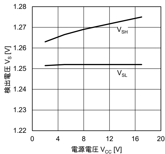
検出電圧 - 電源電圧特性
