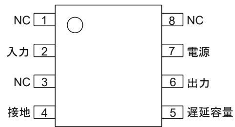
(上面図)
