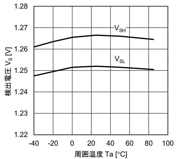
検出電圧 - 周囲温度特性
