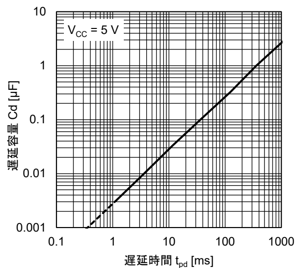
遅延容量 - 遅延時間特性
