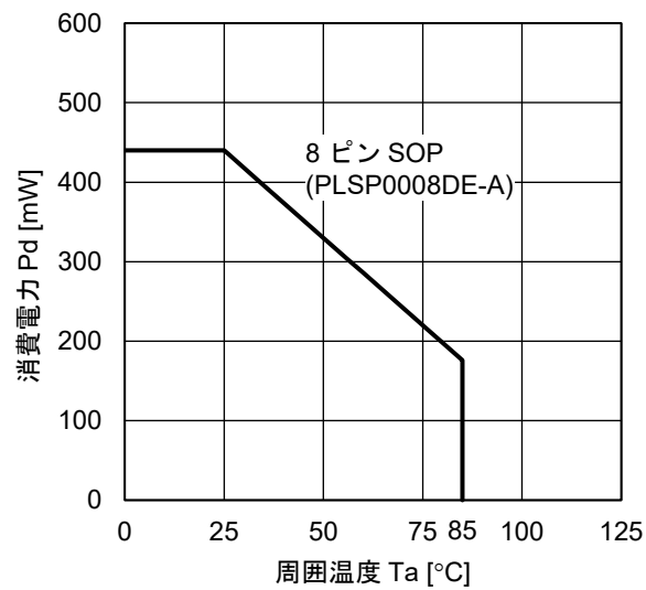
熱低減曲線
