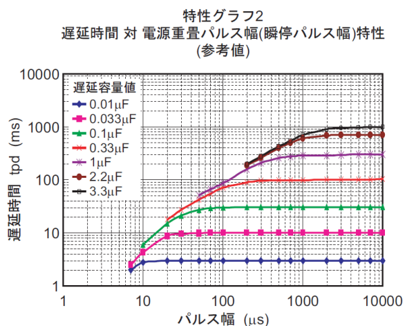
特性グラフ
