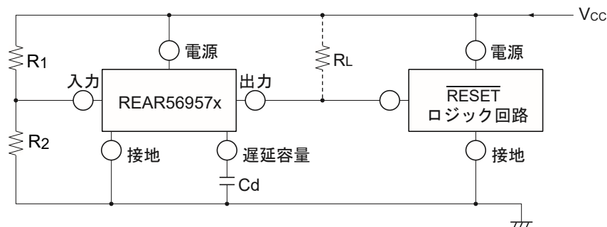
REAR56957 のリセット回路への応用
