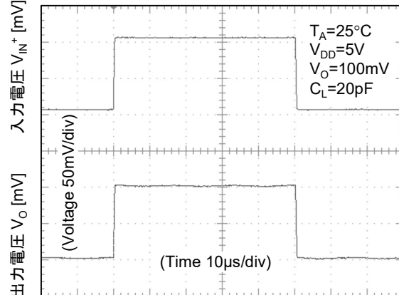
小振幅過渡応答特性
