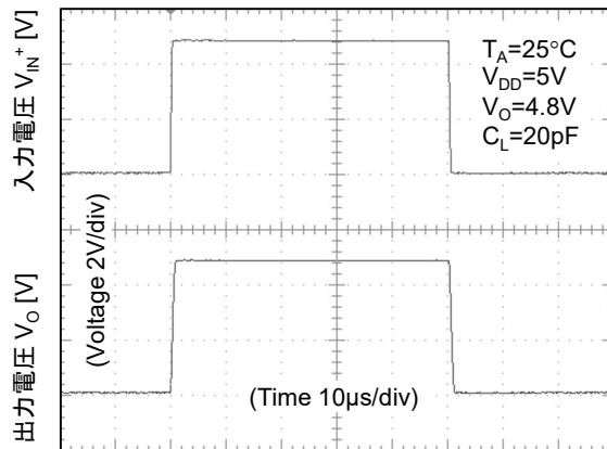
大振幅過渡応答特性
