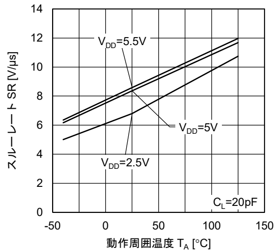
SR - T_A 特性 (出力立ち下がり)
