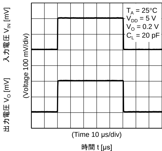
小振幅過渡応答特性
