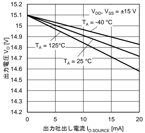
V_O - I_{O\text{SOURCE}} 特性
