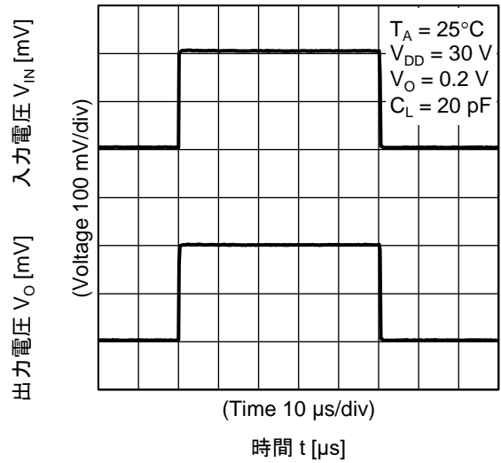
小振幅過度応答特性
