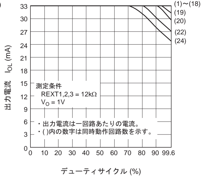
デューティサイクル-出力電流特性
