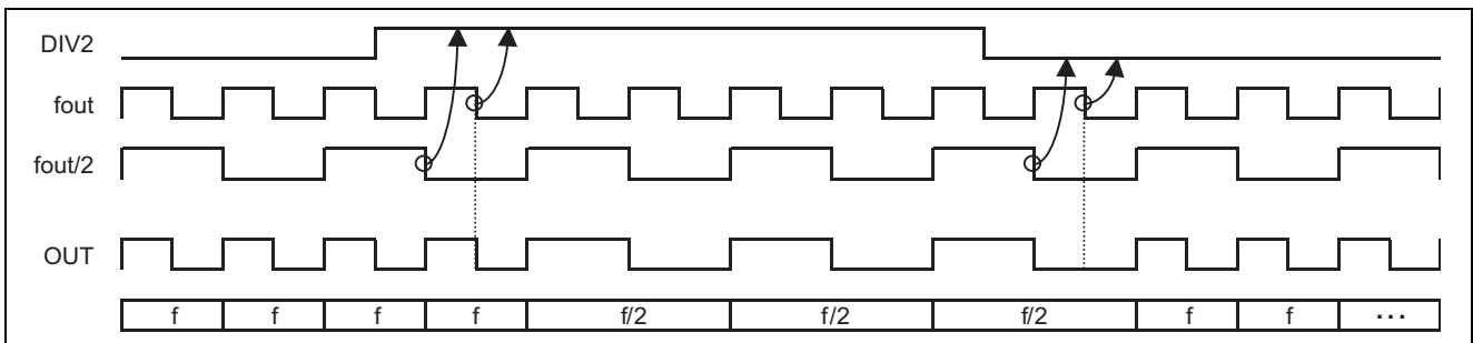
図 2 Timing chart
