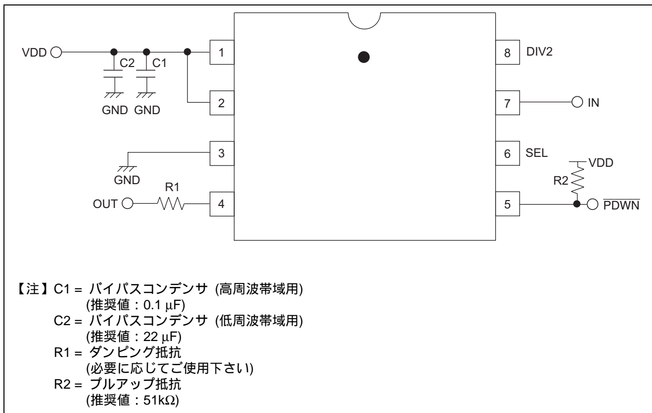
図3 推奨外付け回路
