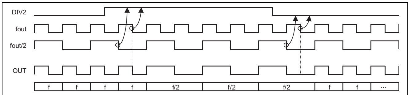
図 2 Timing chart
