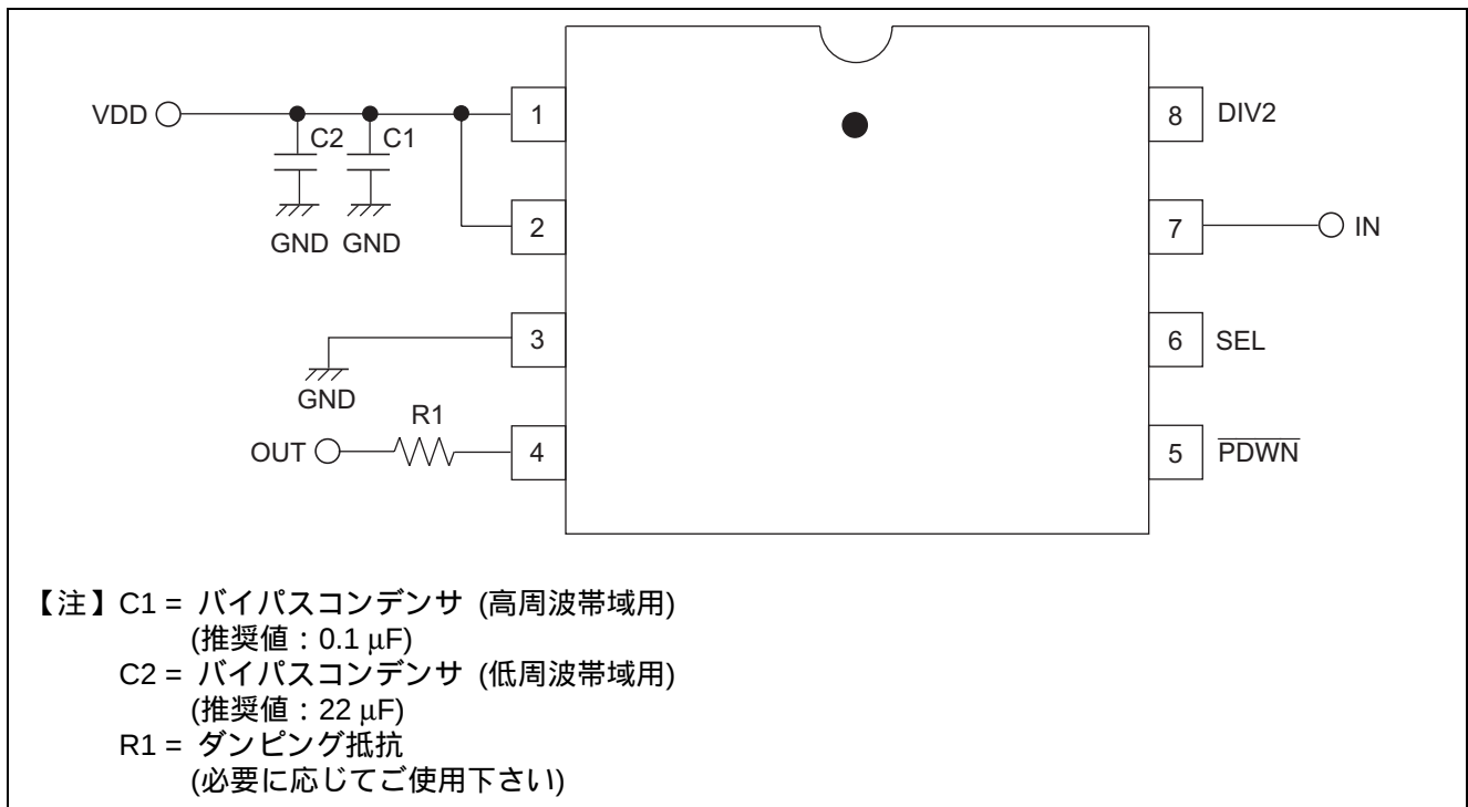
図 3 推奨外付け回路
