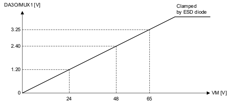
Figure 6.5-6 DA3O / MUX1 と VM 電圧の関係
