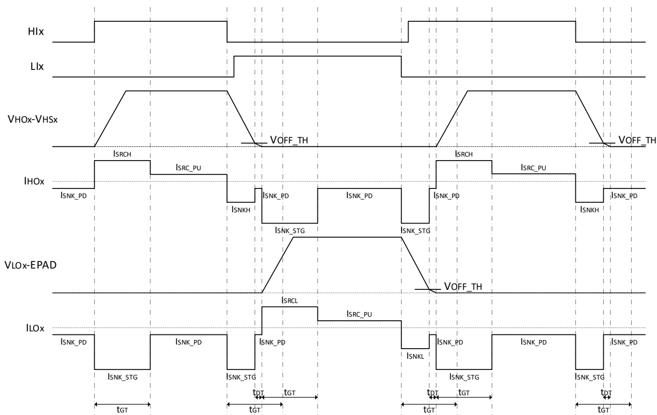
Figure 6.4-3 HI/LI によるデッドタイムが比較的に短い場合の 3 相 HI/LI モードのゲートドライブタイミング
