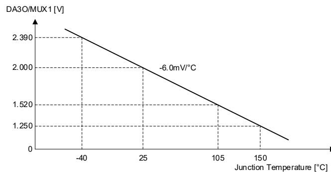
Figure 6.5-7 DA3O / MUX1 とジャンクション温度との関係
