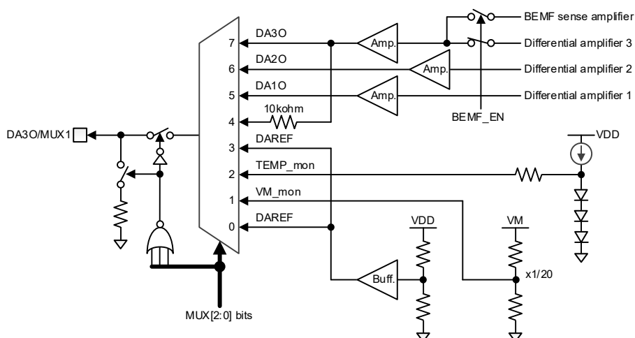
Figure 6.5-5 DA3O / MUX1 端子用アナログマルチプレクサのブロック図
