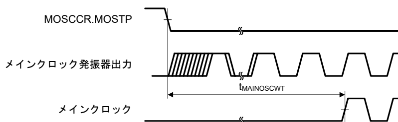
図 2.4 メインクロック発振開始タイミング
