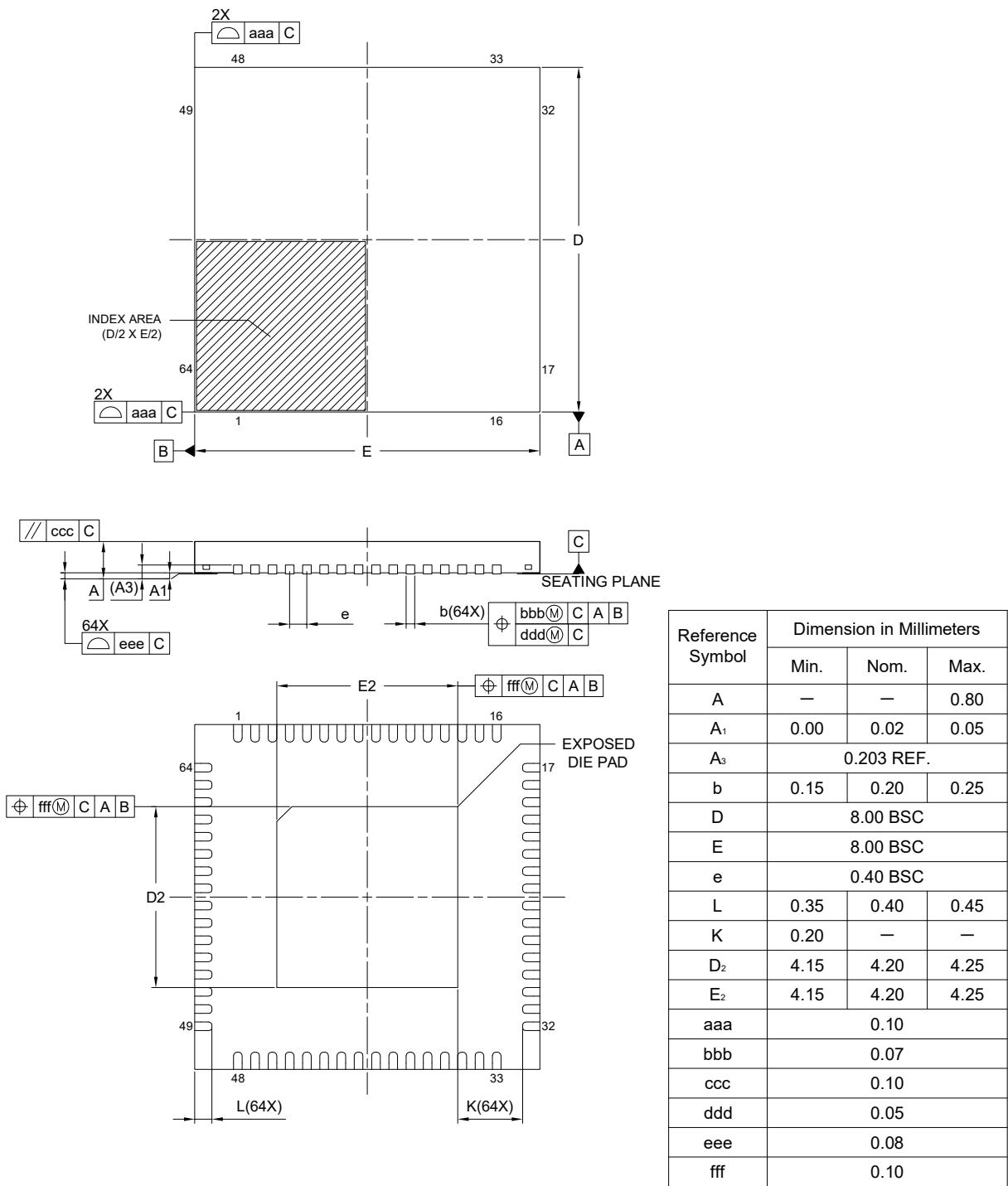
図 A2.3 QFN 64 ピン
