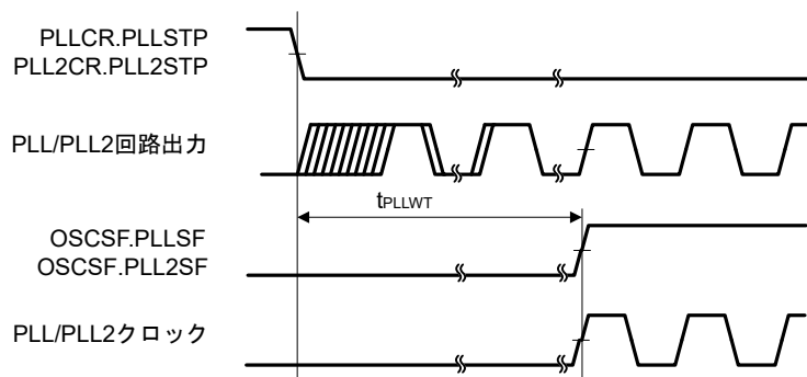
図 2.6 PLL/PLL2 クロック発振開始タイミング
