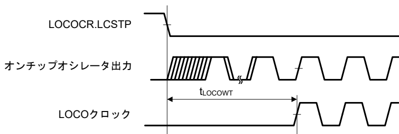
図 2.5 LOCO クロック発振開始タイミング
