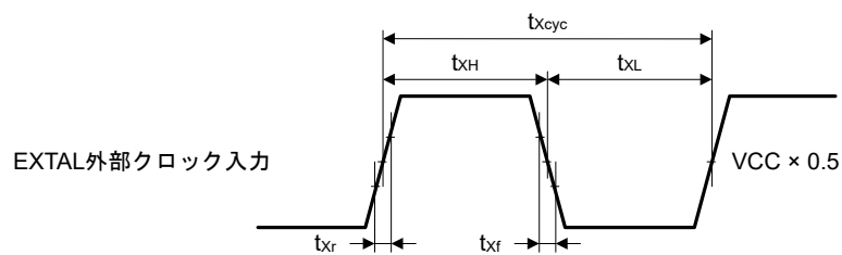
図 2.3 EXTERNAL 外部クロック入力タイミング
