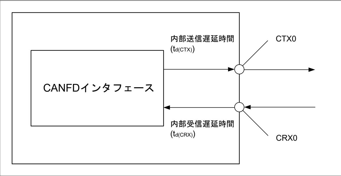
図 2.49 CANFD インタフェース条件
