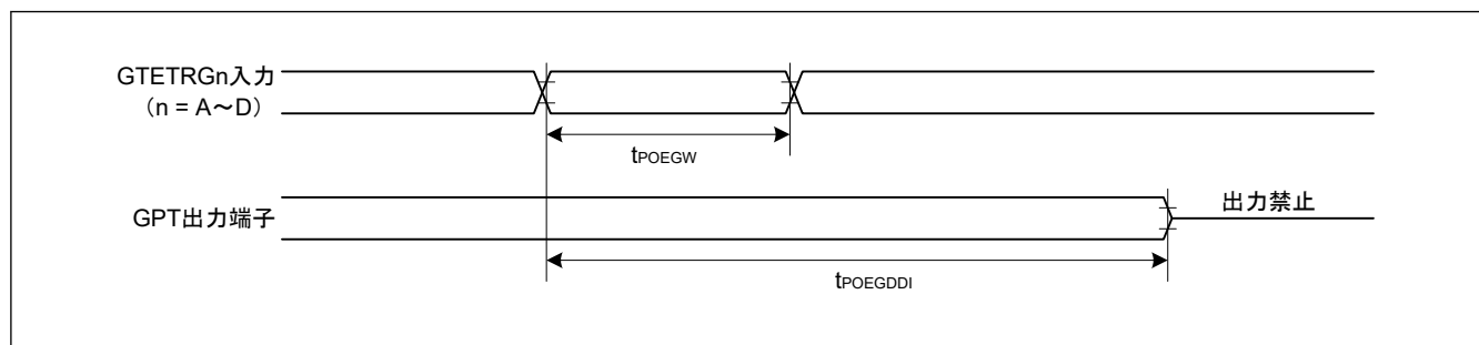
図 2.21 GTETR Gn 端子の入力レベル検出に直接対応した POEG の出力禁止時間
