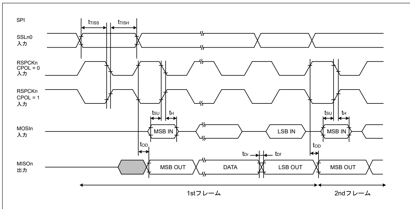
図 2.46 フレーム間の遅延がない送信における TI SSP スレーブの SPI タイミング
