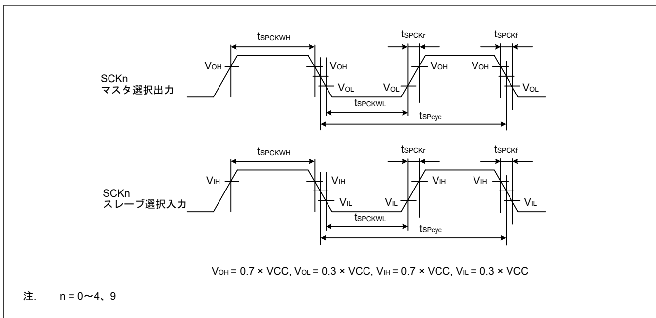
図 2.33 SCI 簡易 SPI モードクロックタイミング
