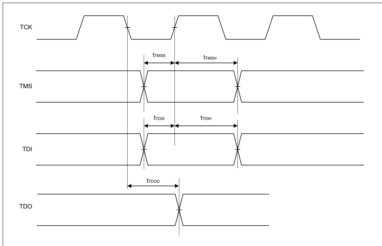
図 2.64 JTAG 入出力タイミング
