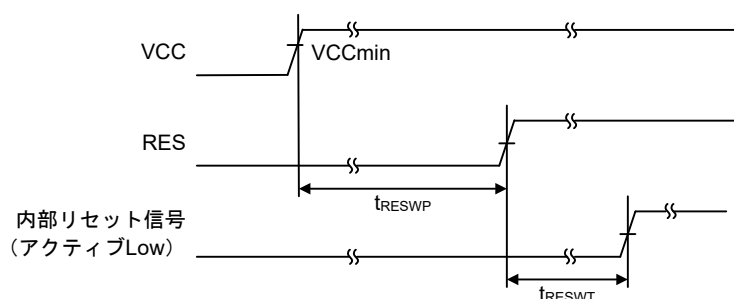
図 2.7 VCC が V_{POR} 電圧しきい値を超える条件下での RES 端子入力タイミグ
