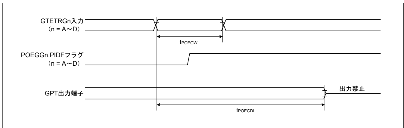
図 2.16 GTETR Gn 端子の入力レベル検出に対応した検出フラグによる POEG の出力禁止時間
