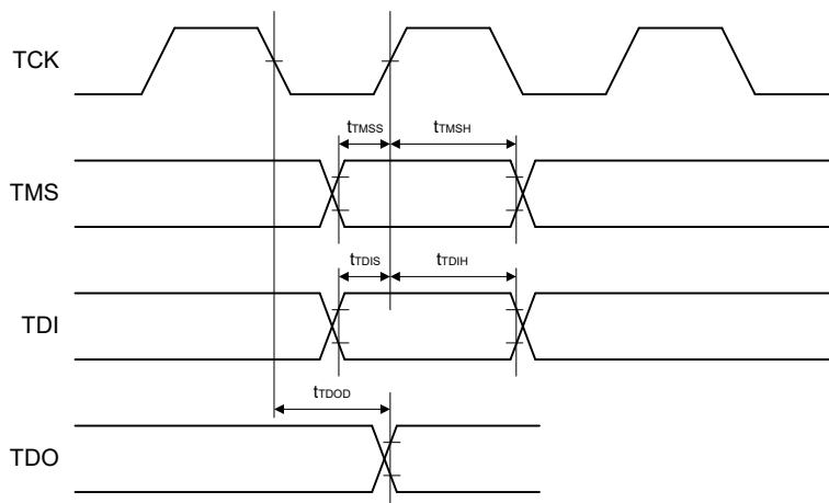
図 2.61 バウンダリスキャン入出力タイミング
