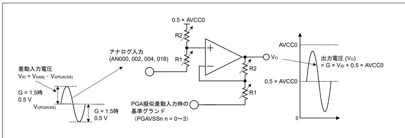
図 2.53 PGA 疑似差動設定時の入出力信号レベル
