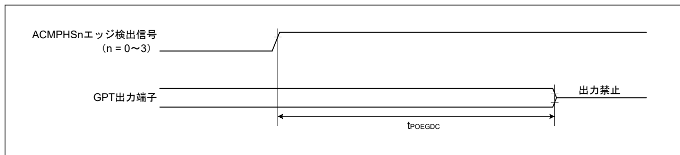
図 2.18 ACMPHS からのエッジ検出信号に対応した POEG の出力禁止時間
