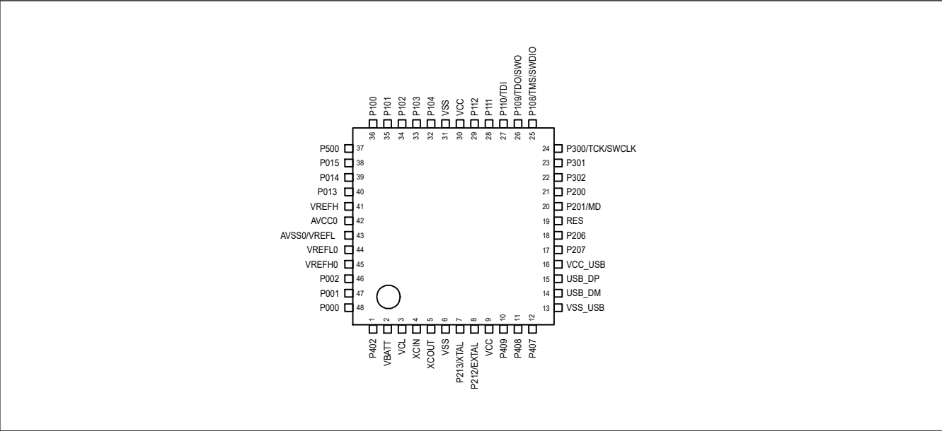
図 1.5 48 ピン LQFP のピン配置
