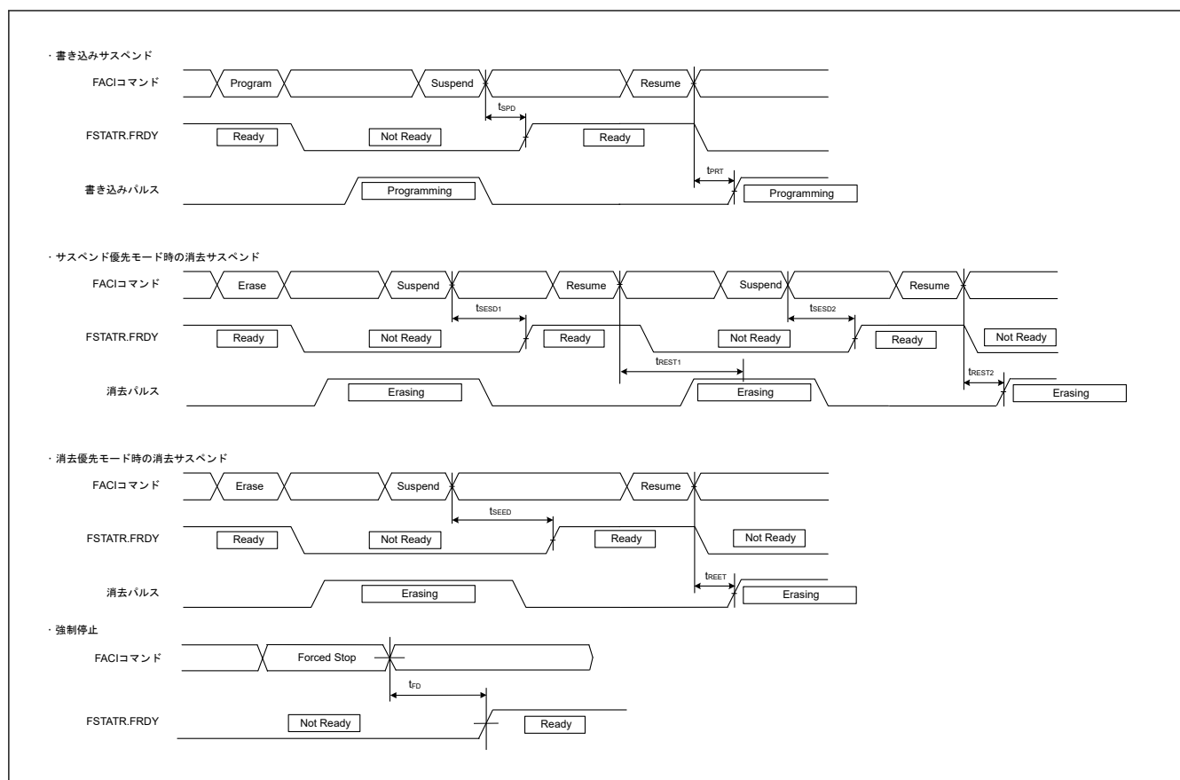
図 2.63 フラッシュメモリのプログラム/イレースのサスペンドタイミングと強制停止タイミング
