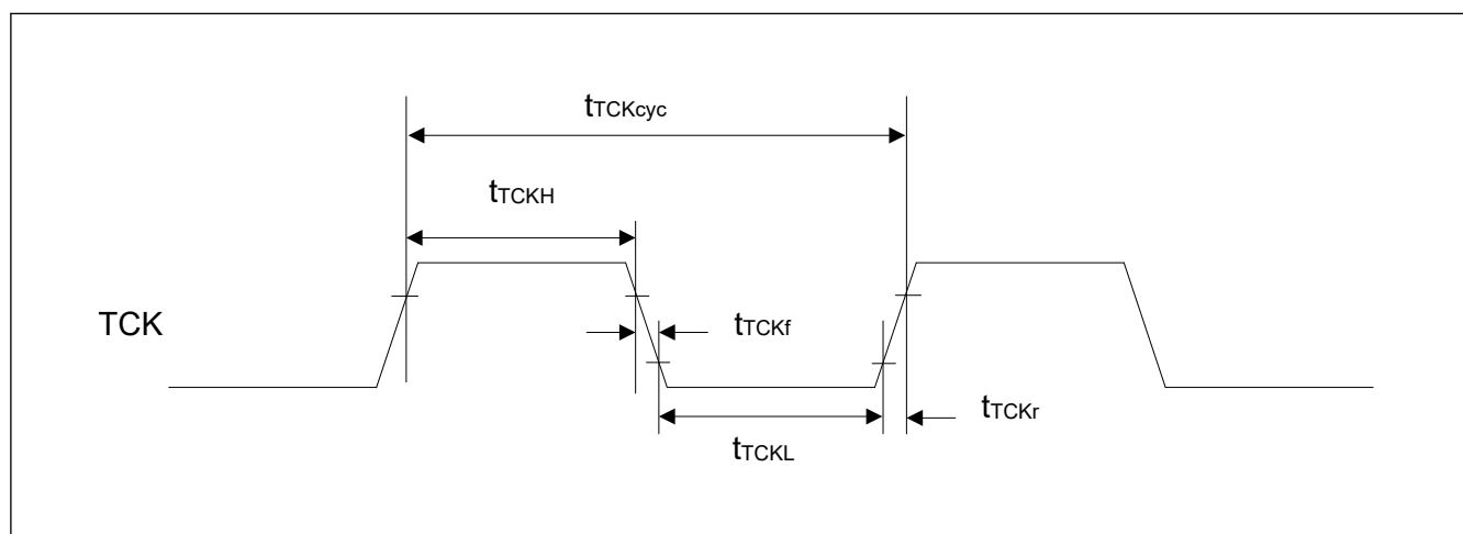
図 2.67 JTAG TCK タイミング
