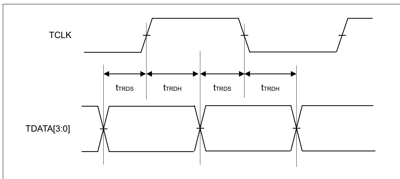
図 2.72 ETM 出力タイミング
