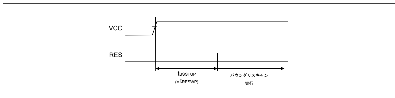
図 2.66 バウンダリスキャン回路起動タイミング
