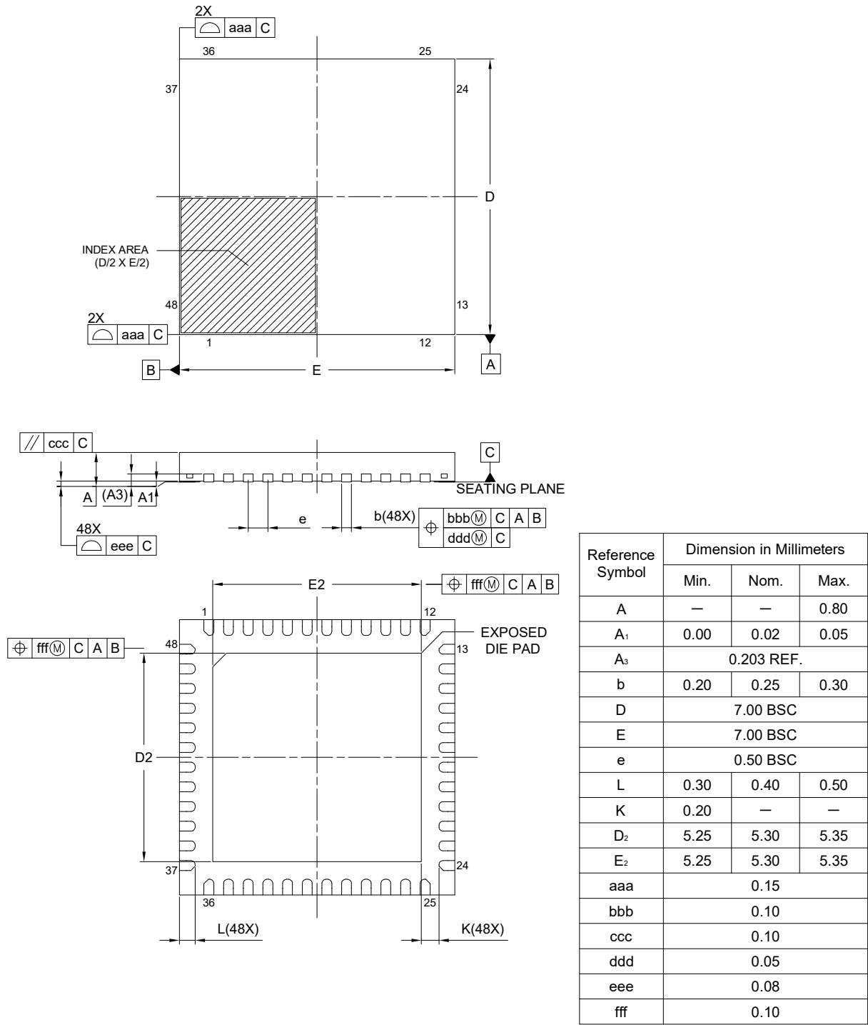
図 A2.4 QFN 48 ピン
