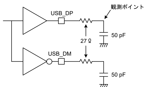
図 2.53 フルスピードモードにおける測定回路
