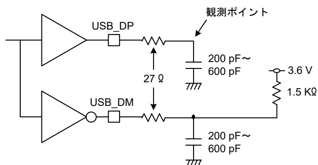
図 2.51 Low-speed モードにおける測定回路
