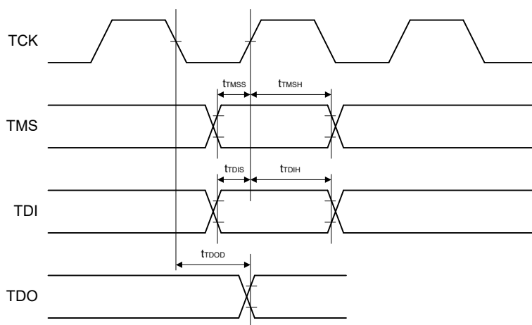
図 2.65 バウンダリスキャン入出力タイミング
