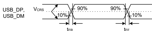
図 2.52 フルスピードモードにおける USB_DP、USB_DM の出力タイミング
