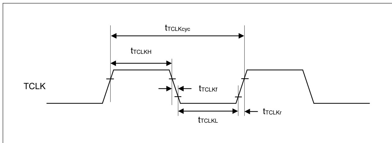
図 2.71 ETM TCLK タイミング
