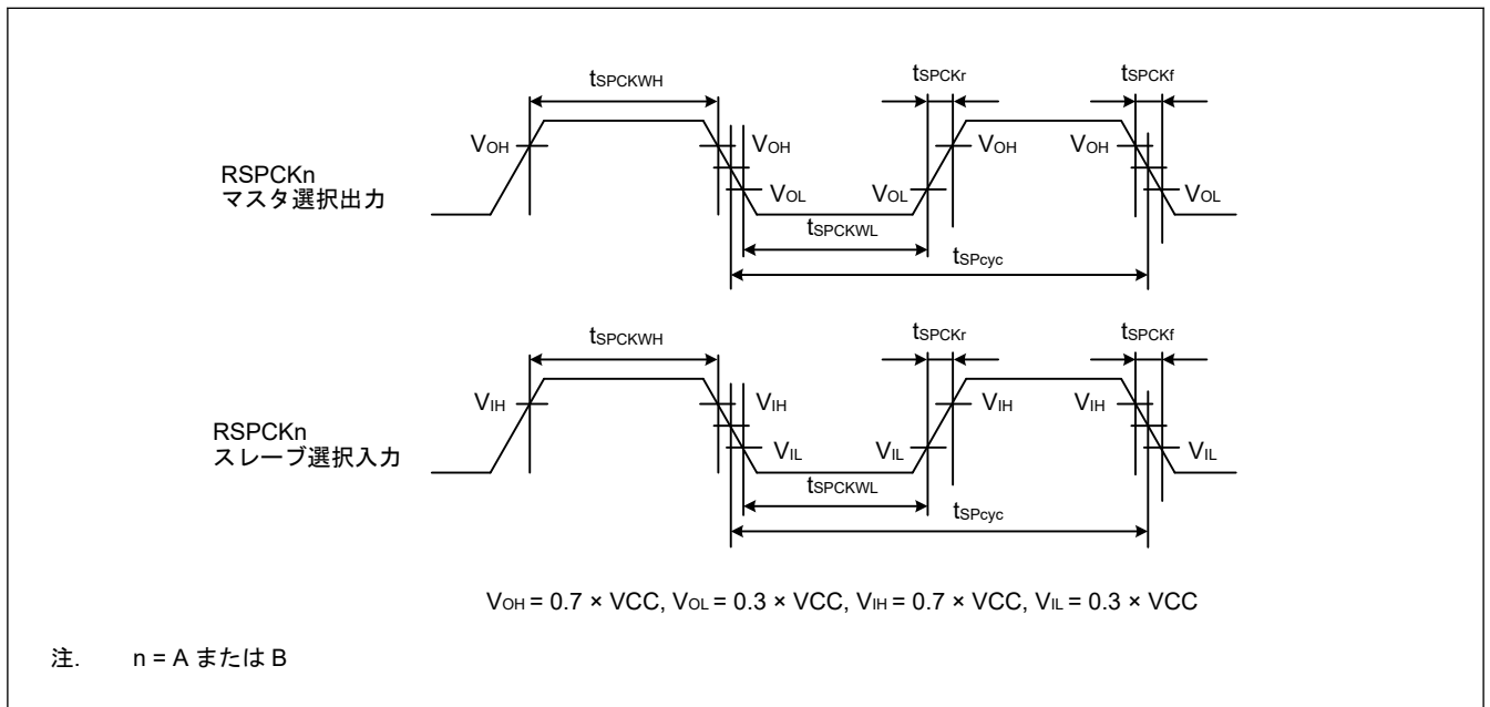
図 2.31 SPI クロックタイミング
