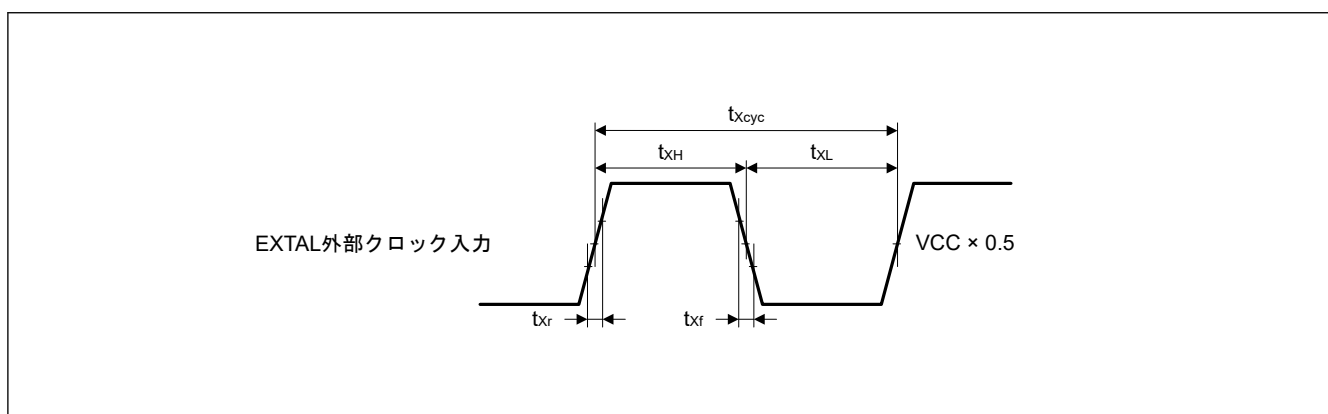
図 2.6 EXTERNAL 外部クロック入力タイミング
