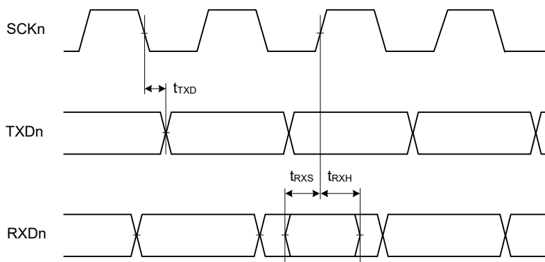
図 2.24 クロック同期式モードにおける SCI 入出力タイミング
