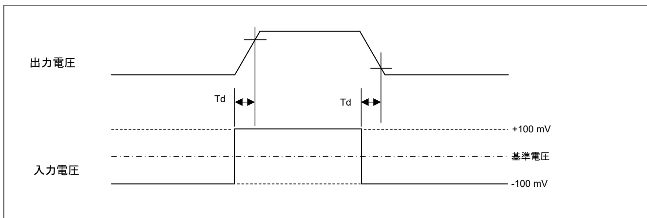
図 2.70 出力遅延時間
