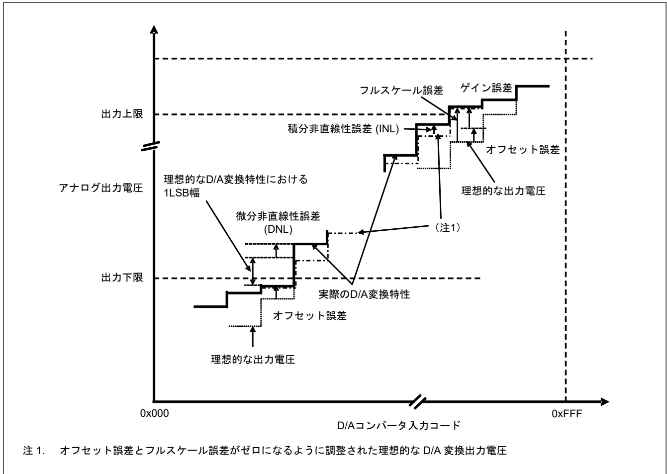
図 2.63 D/A コンバータ 特性用語の解説図
