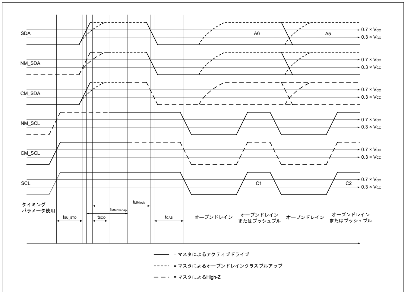
図 2.51 I3C タイミング (オーブンドレインタイミングパラメータ)
